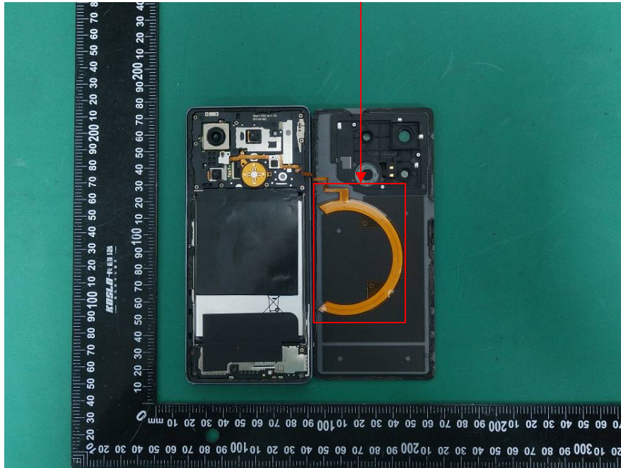
NFC ANT
