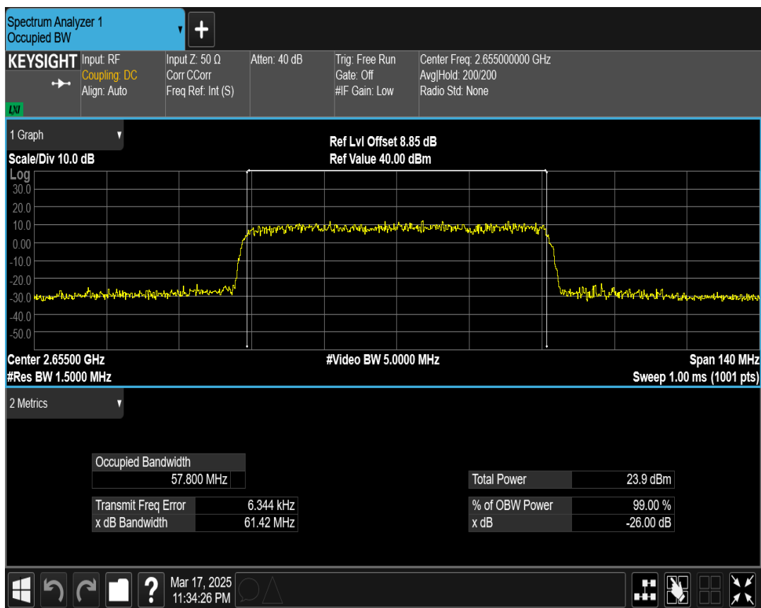
n41 SCS=30kHz CP_QPSK BW=70MHz Channel=531000 RB=189@0
