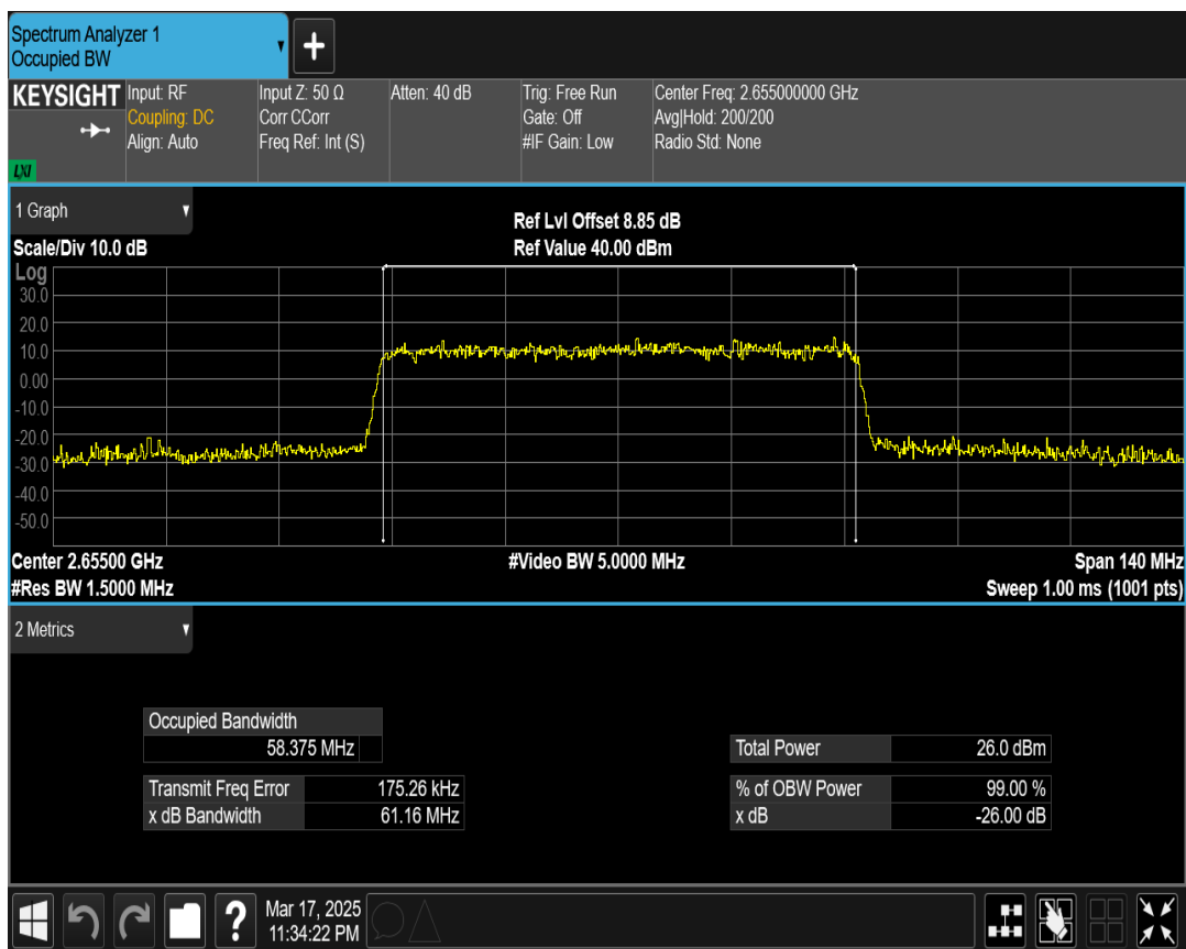
n41 SCS=30kHz DFT_QAM256 BW=70MHz Channel=531000 RB=180@0
