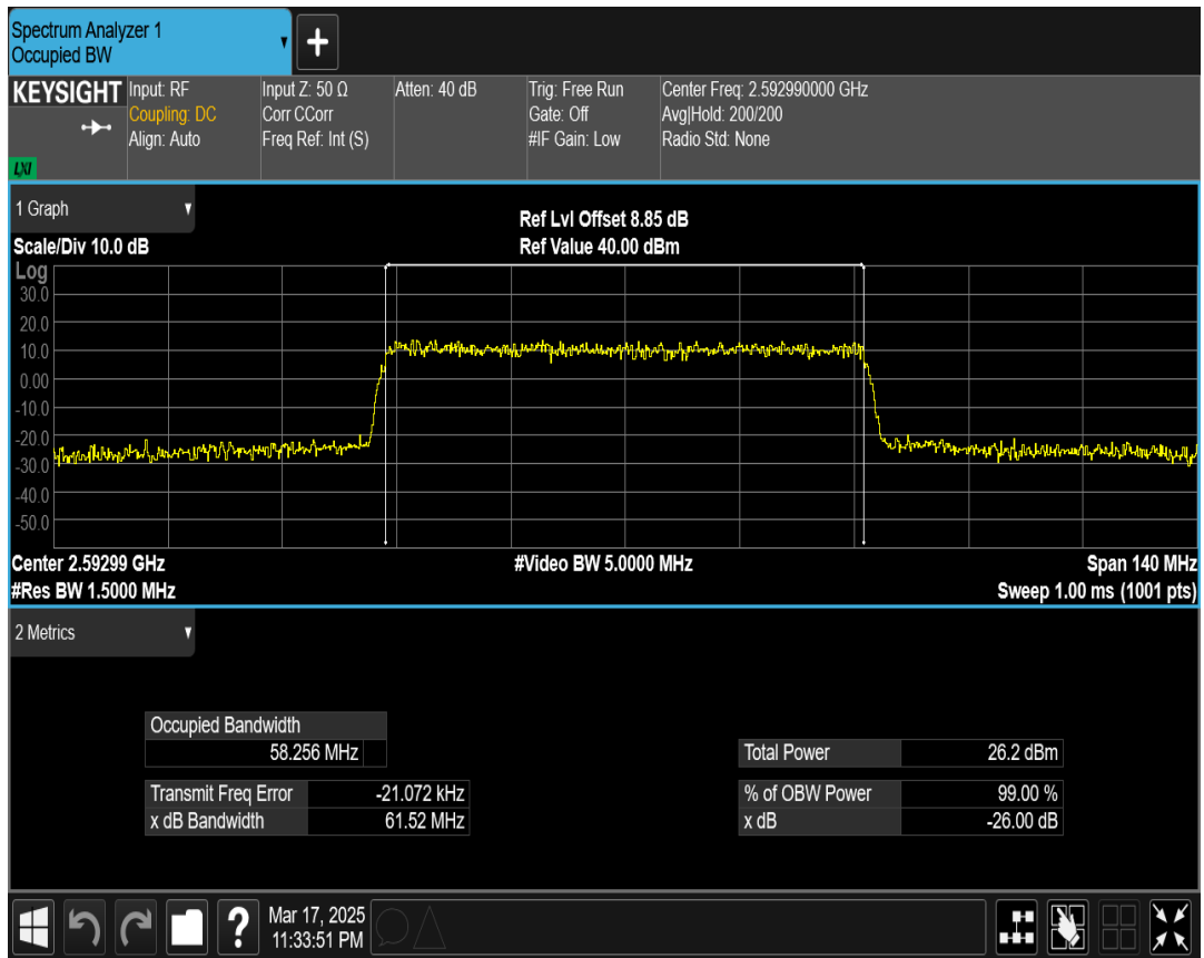
n41 SCS=30kHz DFT_QAM256 BW=70MHz Channel=518598 RB=180@0
