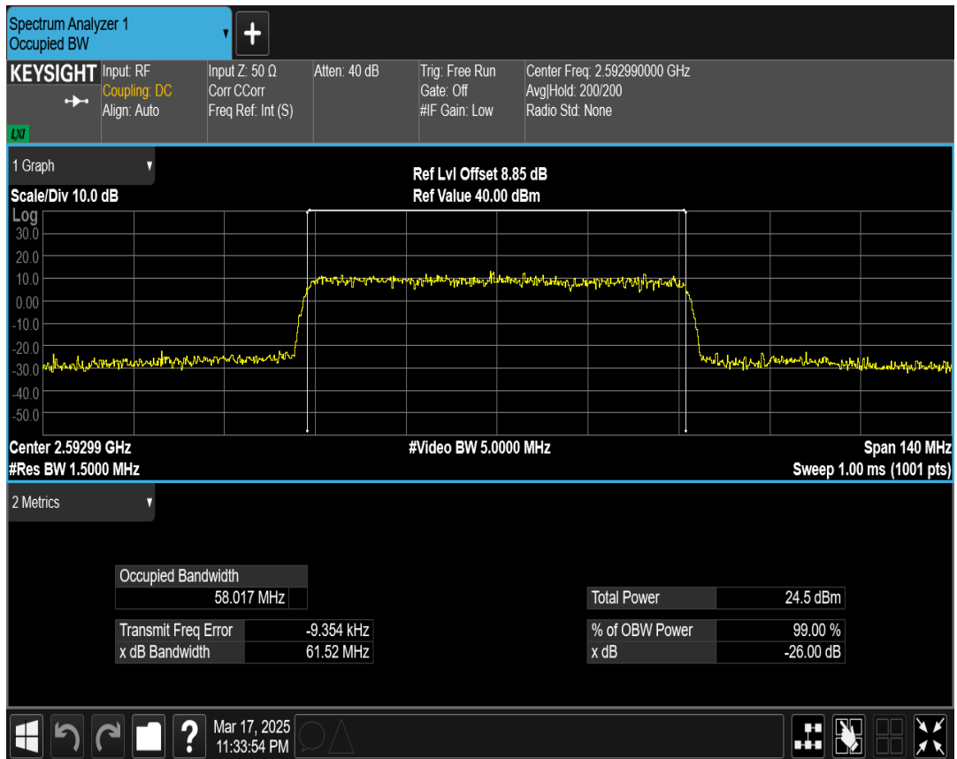
n41 SCS=30kHz CP_QPSK BW=70MHz Channel=518598 RB=189@0
