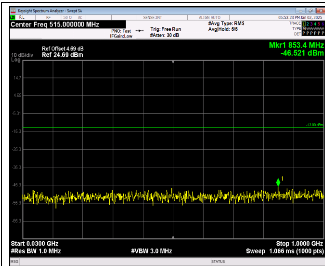
Band66-20MHz-QPSK-132072-1RB#0-Range1:30~1000MHz
