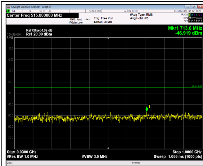
Band41-5MHz-QPSK-41565-1RB#0-Range1:30~100 0MHz
