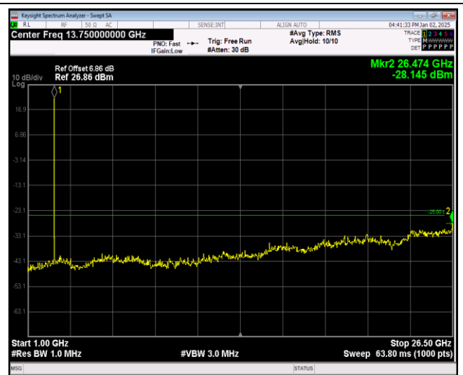
Band41-5MHz-QPSK-41565-1RB#0-Range2:1000~2 6500MHz
