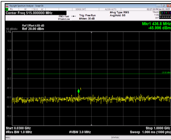
Band7-20MHz-QPSK-20850-1RB#0-Range1:30~100 OMHz
