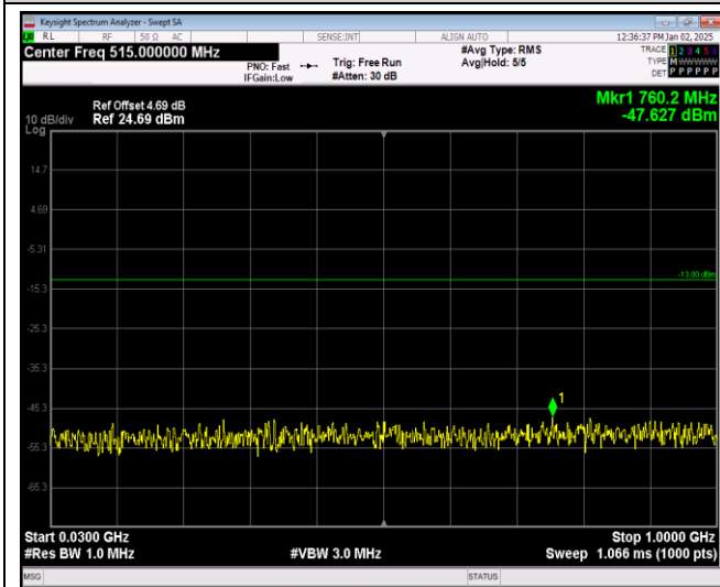
Band4-1.4MHz-QPSK-20175-1RB#0-Range1:30~100 0MHz
