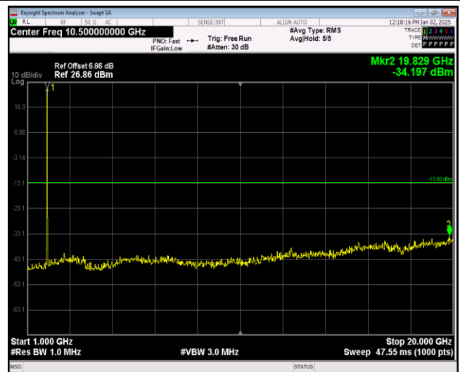
Band2-20MHz-16QAM-18700-1RB#0-Range2:1000~ 20000MHz
