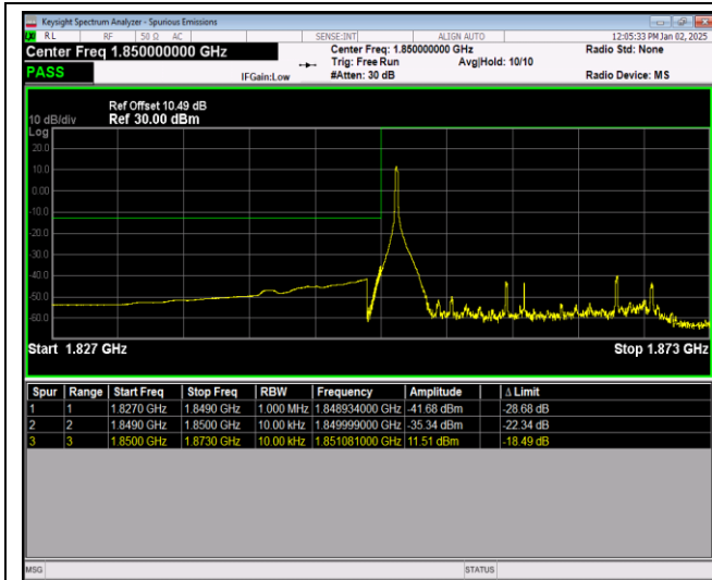
Band2-20MHz-QPSK-18700-100RB#0
