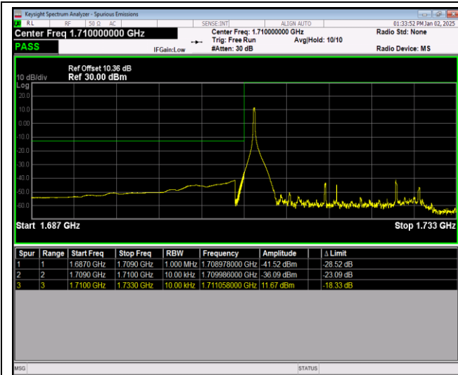
Band4-20MHz-QPSK-20050-100RB#0
