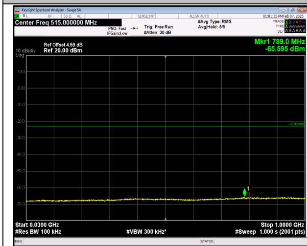
66-66-5MHz-20MHz-16QAM-16QAM-132428-132572-1R B#0-1RB#99-30~1000MHz-PASS
