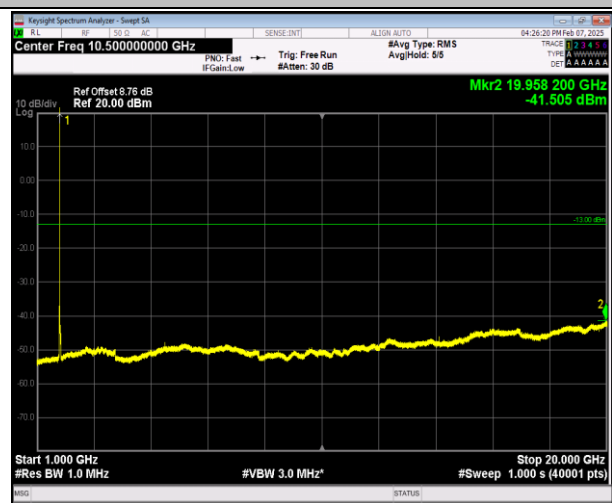
66-66-5MHz-20MHz-QPSK-QPSK-132455-132572-1RB#0- 0RB#0-1000~20000MHz-PASS
