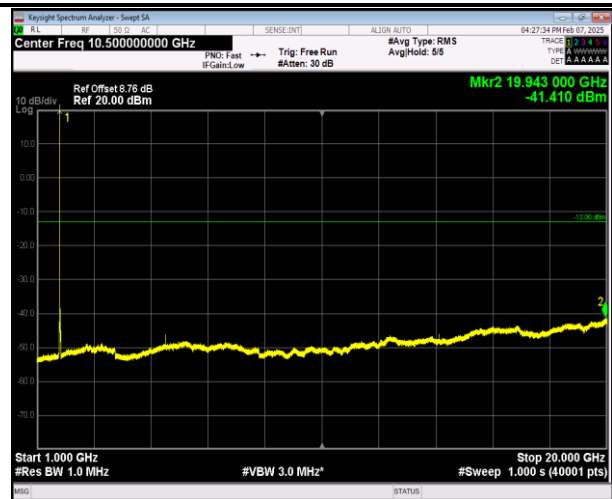
66-66-5MHz-20MHz-QPSK-QPSK-132455-132572-1RB#24 -ORB#0-1000~20000MHz-PASS
