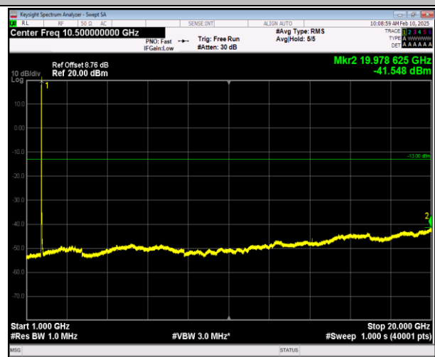
66-66-20MHz-20MHz-16QAM-16QAM-132072-132270-1RB #0-0RB#0-1000~20000MHz-PASS
