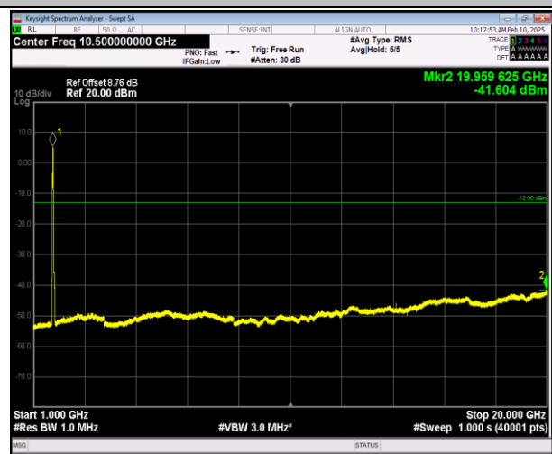
66-66-20MHz-20MHz-16QAM-16QAM-132072-132270-100 RB#0-100RB#0-1000~20000MHz-PASS
