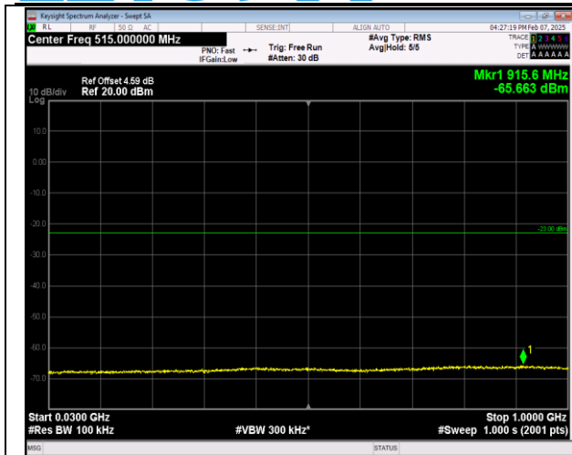
66-66-5MHz-20MHz-QPSK-QPSK-132455-132572-1RB# 24-ORB#0-30~1000MHz-PASS
