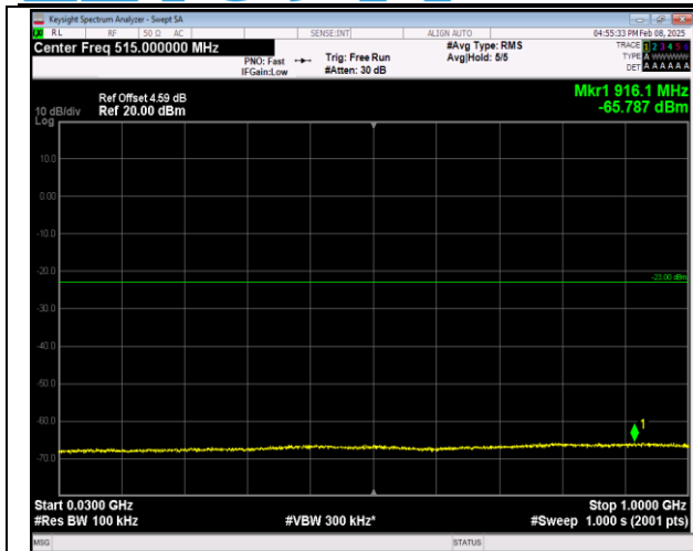
66-66-20MHz-5MHz-QPSK-QPSK-132522-132639-1RB# 99-ORB#0-30~1000MHz-PASS
