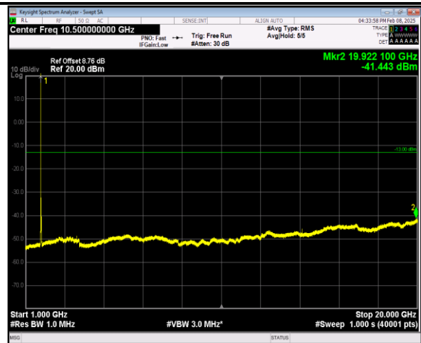
66-66-20MHz-5MHz-16QAM-16QAM-132397-132514-1RB# 0-ORB#0-1000~20000MHz-PASS
