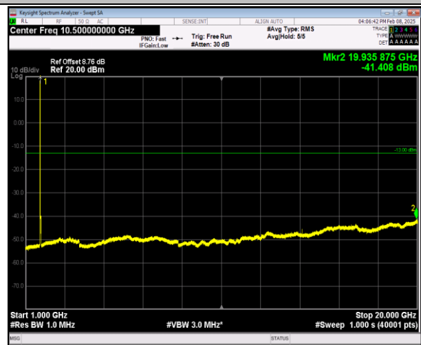
66-66-20MHz-5MHz-16QAM-16QAM-132072-132189-1RB# 0-0RB#0-1000~20000MHz-PASS
