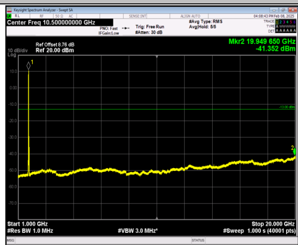
66-66-20MHz-5MHz-QPSK-QPSK-132072-132189-1RB#0- 1RB#24-1000~20000MHz-PASS
