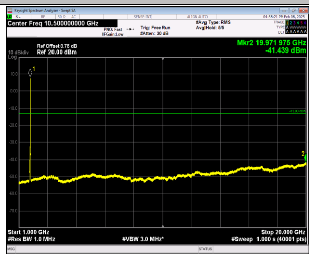
66-66-20MHz-5MHz-QPSK-QPSK-132522-132639-100RB# 0-25RB#0-1000~20000MHz-PASS
