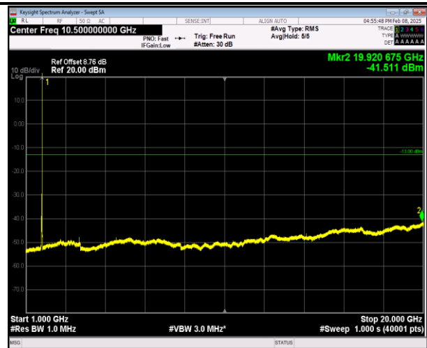
66-66-20MHz-5MHz-QPSK-QPSK-132522-132639-1RB#99 -ORB#0-1000~20000MHz-PASS
