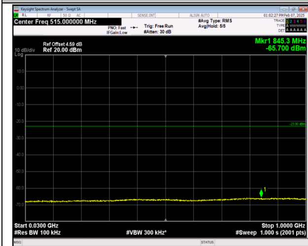
66-66-5MHz-20MHz-QPSK-QPSK-132428-132572-25RB #0-100RB#0-30~1000MHz-PASS
