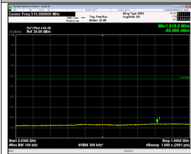
66-66-5MHz-20MHz-QPSK-QPSK-132428-132572-1RB# 24-0RB#0-30~1000MHz-PASS
