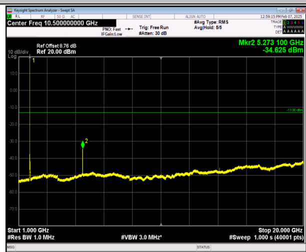
66-66-5MHz-20MHz-QPSK-QPSK-132428-132572-1RB#24 -0RB#0-1000~20000MHz-PASS
