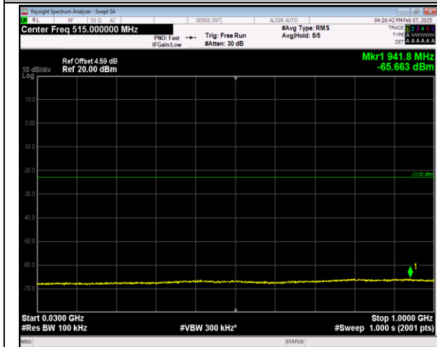
66-66-5MHz-20MHz-16QAM-16QAM-132455-132572-1R B#0-ORB#0-30~1000MHz-PASS
