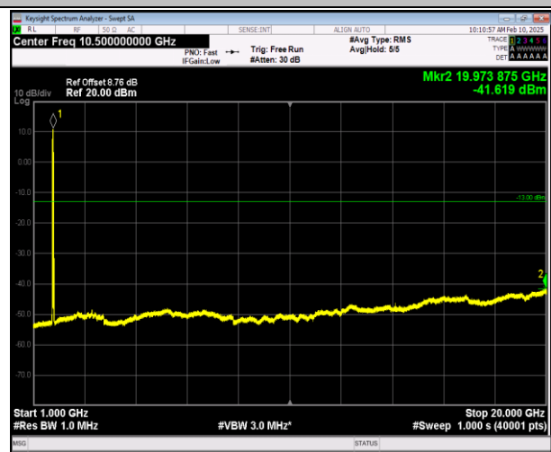
66-66-20MHz-20MHz-QPSK-QPSK-132072-132270-1RB#0 -1RB#99-1000~20000MHz-PASS
