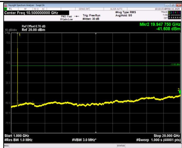
66-66-20MHz-20MHz-16QAM-16QAM-132072-132270-1RB #99-0RB#0-1000~20000MHz-PASS
