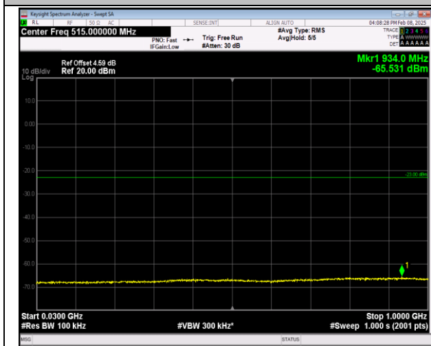
66-66-20MHz-5MHz-QPSK-QPSK-132072-132189-1RB# 0-1RB#24-30~1000MHz-PASS
