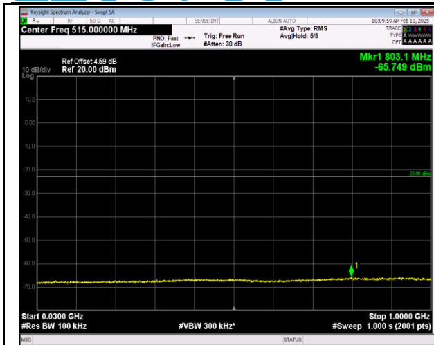
66-66-20MHz-20MHz-16QAM-16QAM-132072-132270-1 RB#99-0RB#0-30~1000MHz-PASS
