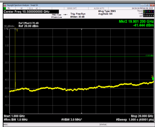
66-66-20MHz-5MHz-QPSK-QPSK-132522-132639-1RB#0- 0RB#0-1000~20000MHz-PASS
