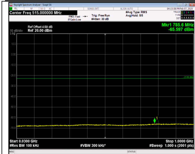
66-66-5MHz-20MHz-QPSK-QPSK-132005-132122-1RB# 0-ORB#0-30~1000MHz-PASS
