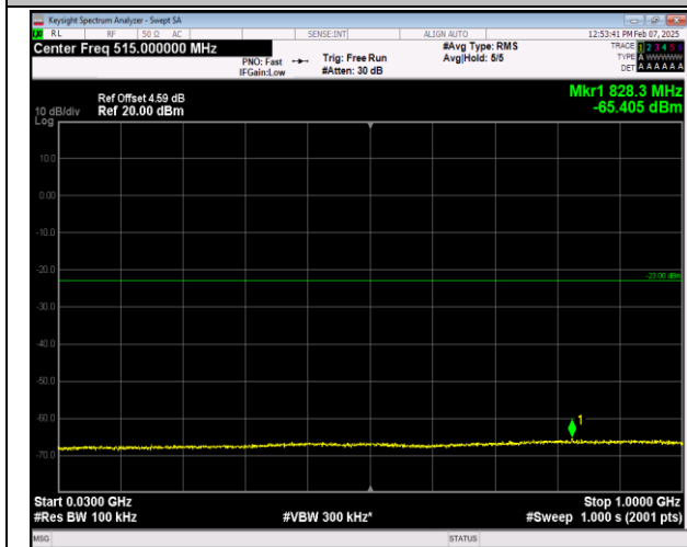
66-66-5MHz-20MHz-QPSK-QPSK-132328-132472-1RB# 0-1RB#99-30~1000MHz-PASS
