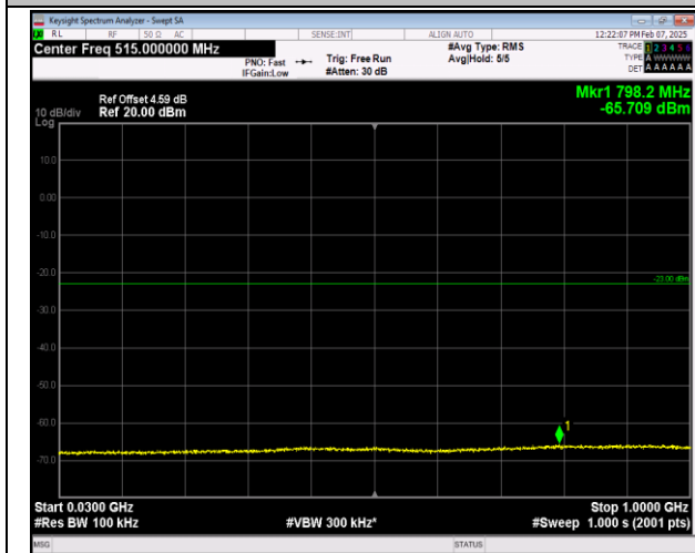
66-66-5MHz-20MHz-QPSK-QPSK-132027-132171-1RB# 0-ORB#0-30~1000MHz-PASS
