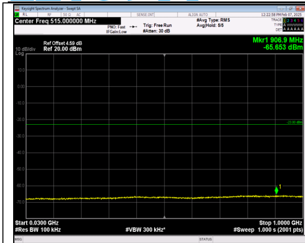
66-66-5MHz-20MHz-16QAM-16QAM-132027-132171-1R B#0-ORB#0-30~1000MHz-PASS
