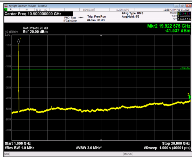
66-66-5MHz-20MHz-QPSK-QPSK-132328-132472-25RB#0 -100RB#0-1000~20000MHz-PASS
