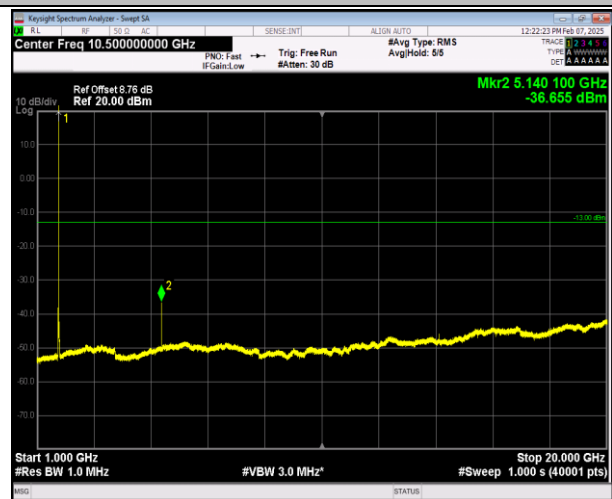
66-66-5MHz-20MHz-QPSK-QPSK-132027-132171-1RB#0- ORB#0-1000~20000MHz-PASS
