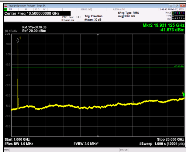
66-66-5MHz-20MHz-QPSK-QPSK-132027-132171-25RB#0 -100RB#0-1000~20000MHz-PASS
