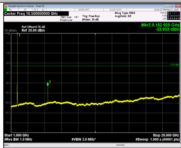
66-66-5MHz-20MHz-QPSK-QPSK-132027-132171-1RB#24 -0RB#0-1000~20000MHz-PASS
