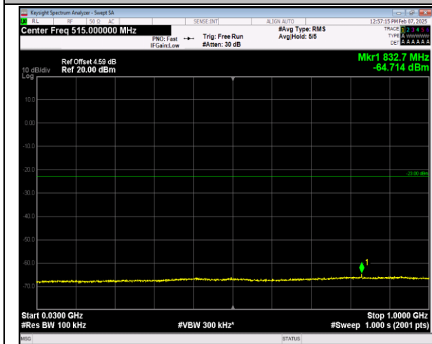
66-66-5MHz-20MHz-QPSK-QPSK-132428-132572-1RB# 0-ORB#0-30~1000MHz-PASS
