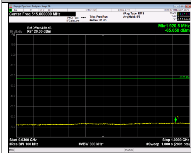
66-66-5MHz-20MHz-QPSK-QPSK-132328-132472-1RB# 0-0RB#0-30~1000MHz-PASS
