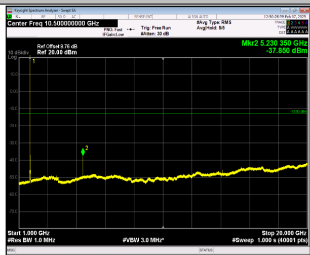
66-66-5MHz-20MHz-QPSK-QPSK-132328-132472-1RB#0- 0RB#0-1000~20000MHz-PASS
