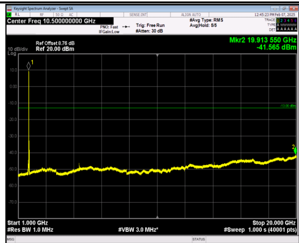
66-66-5MHz-20MHz-QPSK-QPSK-132027-132171-1RB#0- 1RB#99-1000~20000MHz-PASS
