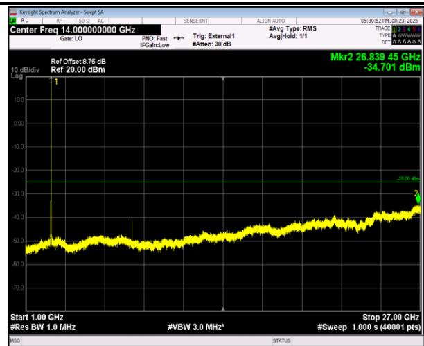
41-41-20MHz-20MHz-QPSK-QPSK-41292-41490-1RB#99- ORB#0-1000~27000MHz-PASS
