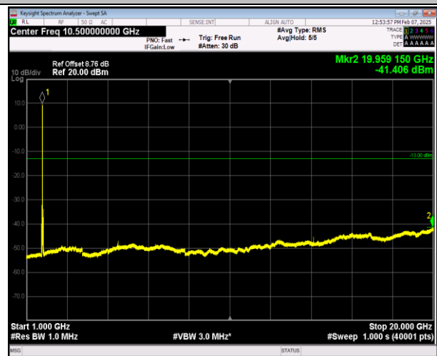
66-66-5MHz-20MHz-QPSK-QPSK-132328-132472-1RB#0- 1RB#99-1000~20000MHz-PASS
