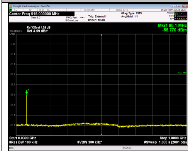
41-41-20MHz-20MHz-QPSK-QPSK-41292-41490-1RB#0 -0RB#0-30~1000MHz-PASS
