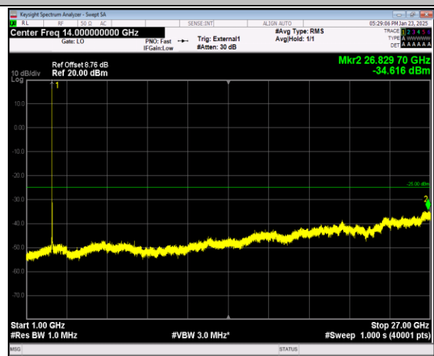
41-41-20MHz-20MHz-QPSK-QPSK-41292-41490-1RB#0-0 RB#0-1000~27000MHz-PASS
