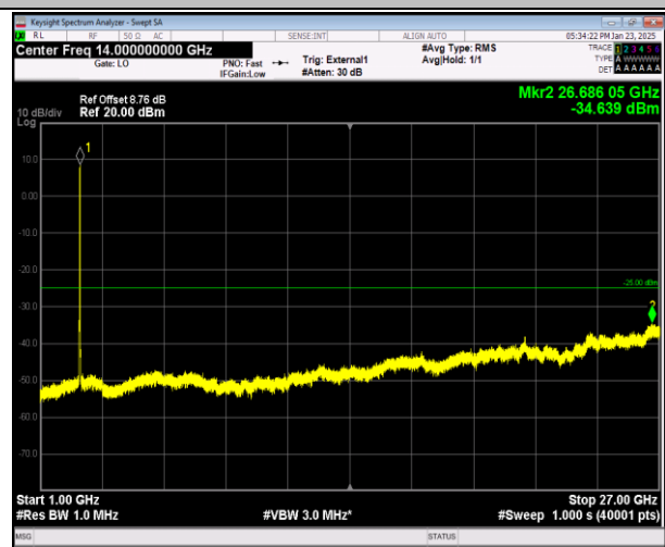
41-41-20MHz-20MHz-QPSK-QPSK-41292-41490-100RB#0 -100RB#0-1000~27000MHz-PASS
