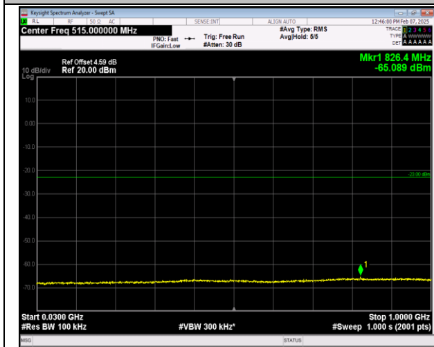
66-66-5MHz-20MHz-16QAM-16QAM-132027-132171-1R B#0-1RB#99-30~1000MHz-PASS
