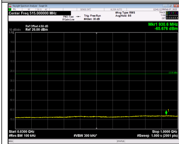
66-66-5MHz-20MHz-QPSK-QPSK-132027-132171-1RB# 24-0RB#0-30~1000MHz-PASS
