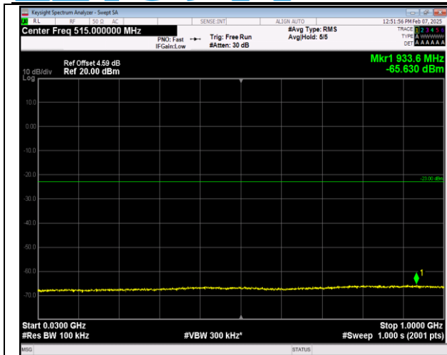
66-66-5MHz-20MHz-QPSK-QPSK-132328-132472-1RB# 24-ORB#0-30~1000MHz-PASS
