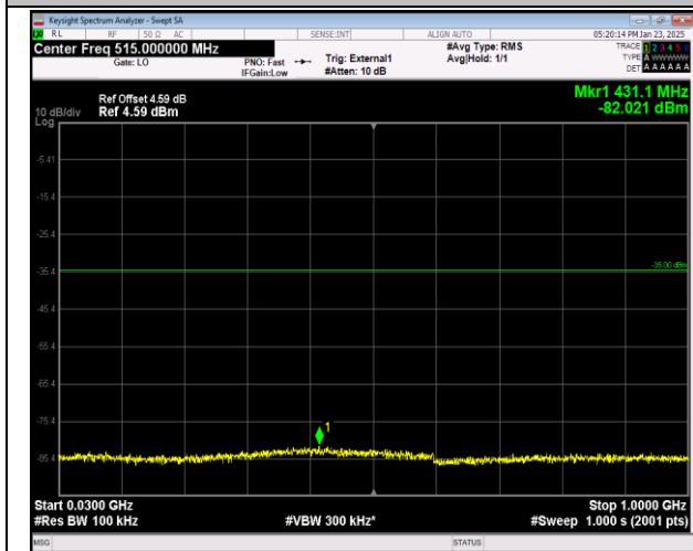
41-41-20MHz-20MHz-QPSK-QPSK-40521-40719-1RB#0 -0RB#0-30~1000MHz-PASS
