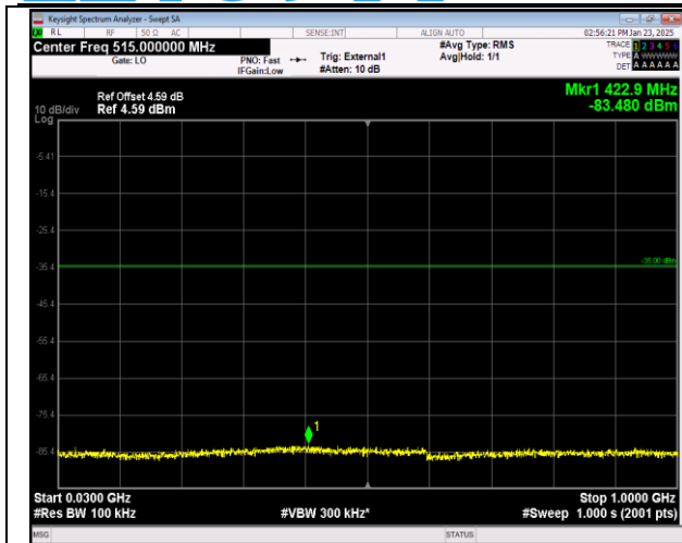
41-41-20MHz-10MHz-QPSK-QPSK-39750-39894-100RB #0-50RB#0-30~1000MHz-PASS
