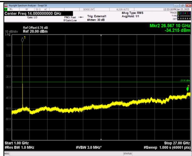
41-41-20MHz-5MHz-QPSK-QPSK-40595-40712-1RB#0-1RB#24-1000~27000MHz-PASS
