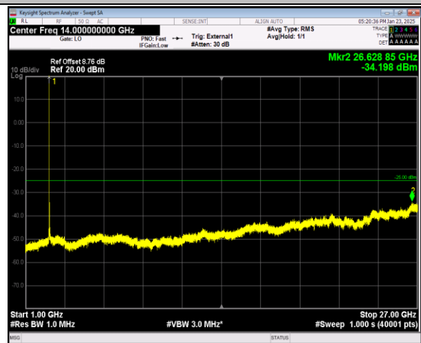
41-41-20MHz-20MHz-QPSK-QPSK-40521-40719-1RB#0-0 RB#0-1000~27000MHz-PASS
