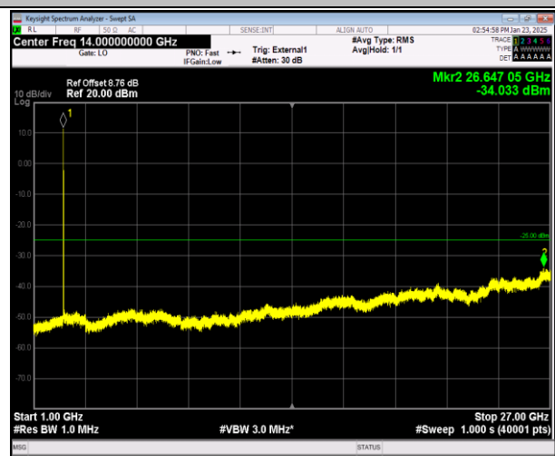
41-41-20MHz-10MHz-QPSK-QPSK-39750-39894-1RB#0-1 RB#49-1000~27000MHz-PASS
