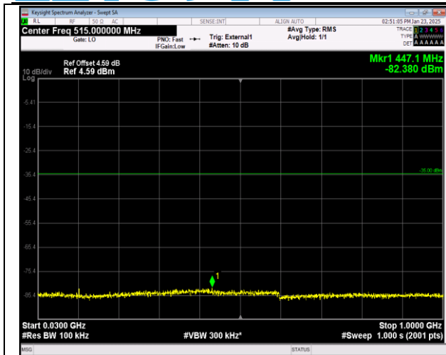
41-41-20MHz-10MHz-QPSK-QPSK-39750-39894-1RB#0 -ORB#0-30~1000MHz-PASS
