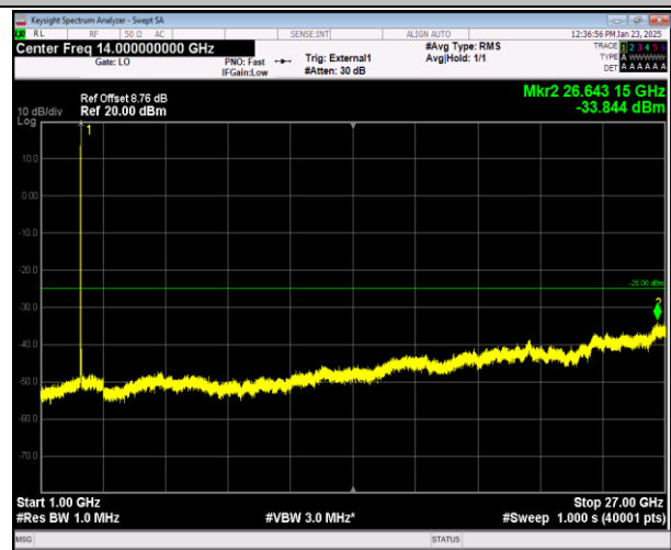
41-41-20MHz-5MHz-QPSK-QPSK-41440-41557-1RB#0-0RB#0-1000~27000MHz-PASS
