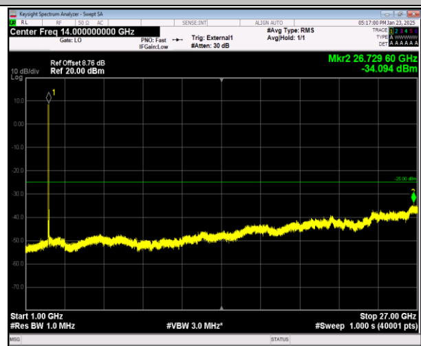
41-41-20MHz-20MHz-QPSK-QPSK-39750-39948-1RB#0-1 RB#99-1000~27000MHz-PASS
