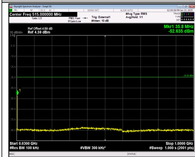
41-41-20MHz-10MHz-QPSK-QPSK-40571-40715-1RB#9 9-0RB#0-30~1000MHz-PASS
