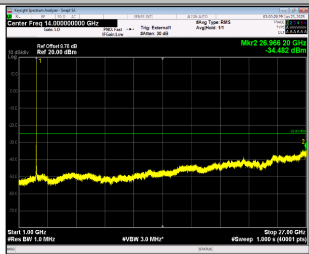
41-41-20MHz-10MHz-QPSK-QPSK-40571-40715-1RB#99- 0RB#0-1000~27000MHz-PASS
