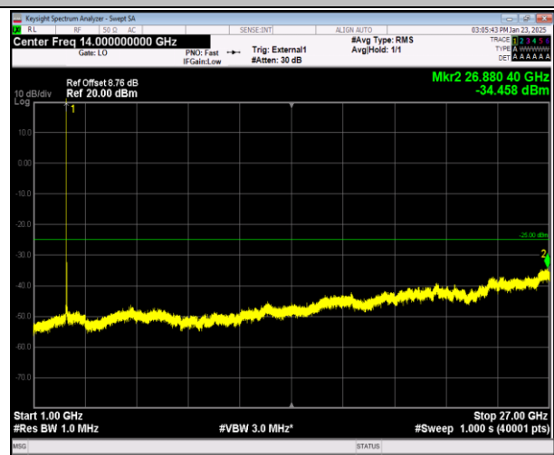
41-41-20MHz-10MHz-QPSK-QPSK-41391-41535-1RB#0-0 RB#0-1000~27000MHz-PASS
