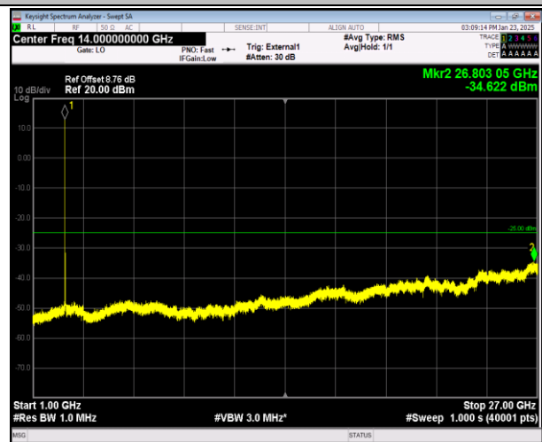
41-41-20MHz-10MHz-QPSK-QPSK-41391-41535-1RB#0-1 RB#49-1000~27000MHz-PASS
