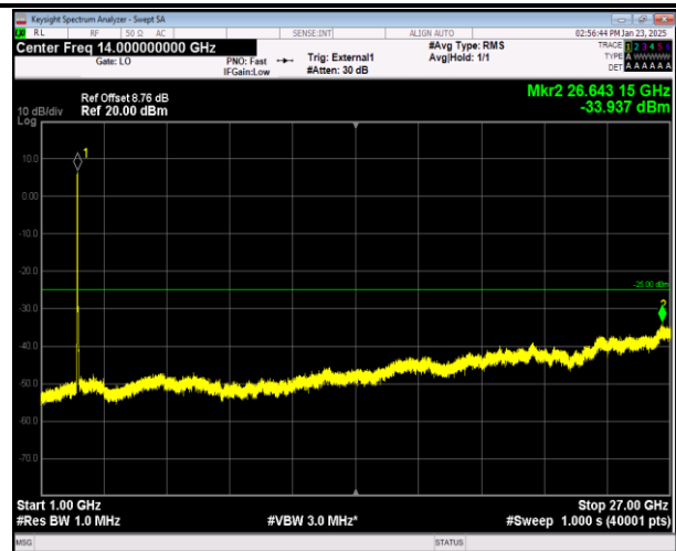
41-41-20MHz-10MHz-QPSK-QPSK-39750-39894-100RB#0 -50RB#0-1000~27000MHz-PASS
