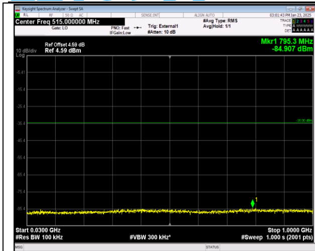
41-41-20MHz-10MHz-QPSK-QPSK-40571-40715-1RB#0 -1RB#49-30~1000MHz-PASS
