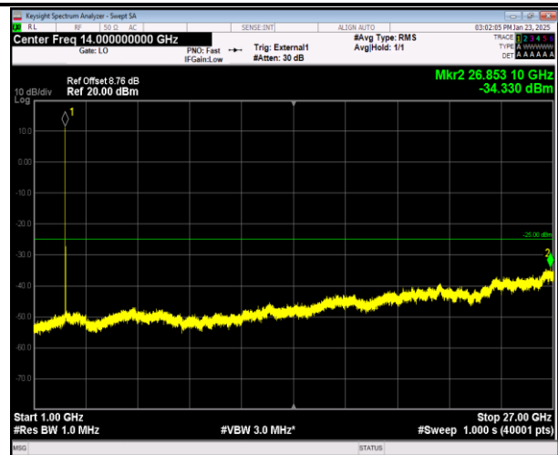
41-41-20MHz-10MHz-QPSK-QPSK-40571-40715-1RB#0-1 RB#49-1000~27000MHz-PASS
