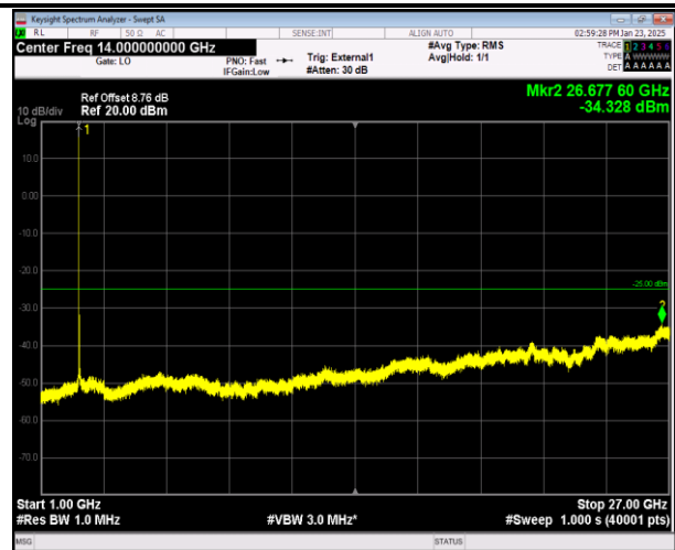
41-41-20MHz-10MHz-16QAM-16QAM-40571-40715-1RB#0 -ORB#0-1000~27000MHz-PASS
