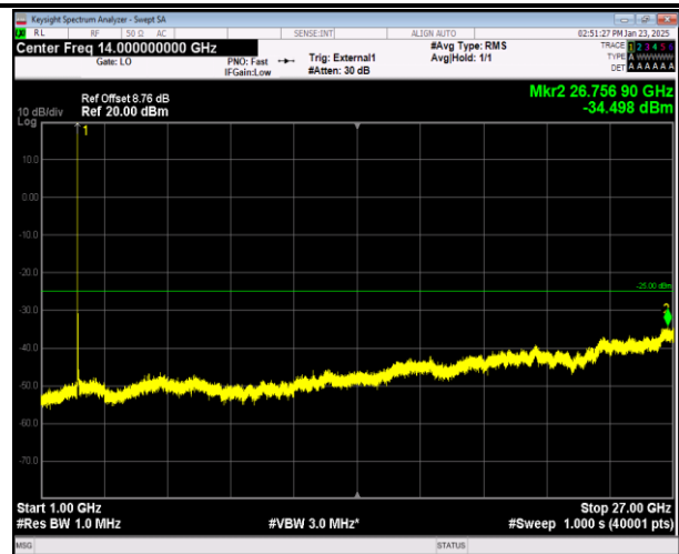
41-41-20MHz-10MHz-QPSK-QPSK-39750-39894-1RB#0-0 RB#0-1000~27000MHz-PASS
