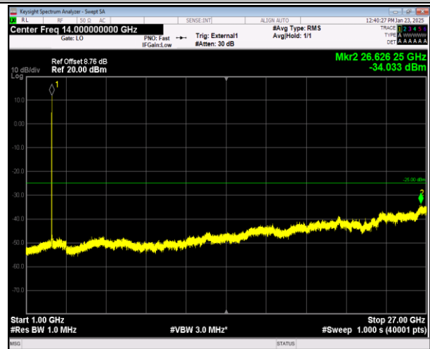
41-41-20MHz-5MHz-QPSK-QPSK-41440-41557-1RB#0-01RB#24-1000~27000MHz-PASS
