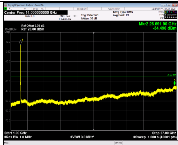
41-41-20MHz-5MHz-QPSK-QPSK-39750-39867-100RB#0- 25RB#0-1000~27000MHz-PASS
