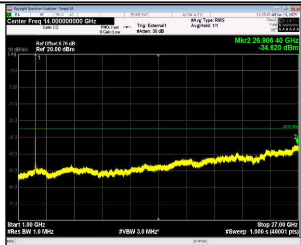
38-38-20MHz-20MHz-QPSK-QPSK-37952-38150-1RB#99- ORB#0-1000~27000MHz-PASS
