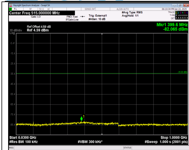
41-41-5MHz-20MHz-QPSK-QPSK-39683-39800-1RB#0-0RB#0-30~1000MHz-PASS
