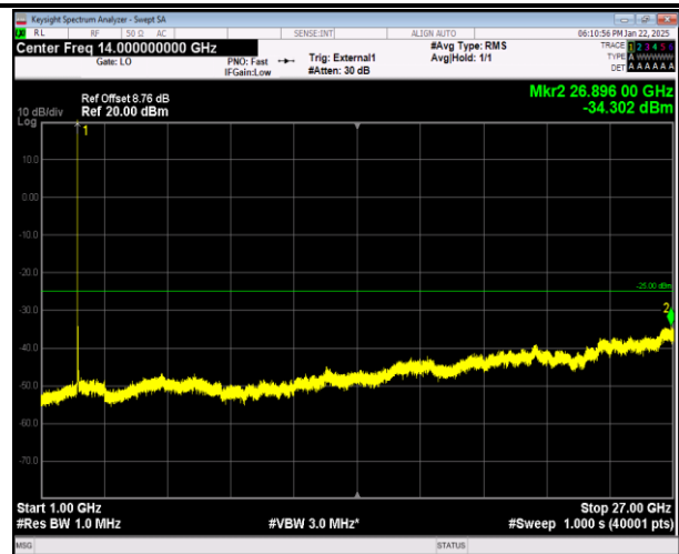
41-41-5MHz-20MHz-QPSK-QPSK-39683-39800-1RB#0-0RB#0-1000~27000MHz-PASS
