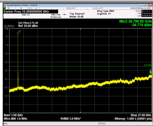
38-38-20MHz-20MHz-16QAM-16QAM-37901-38099-1RB#0 -1RB#99-1000~27000MHz-PASS
