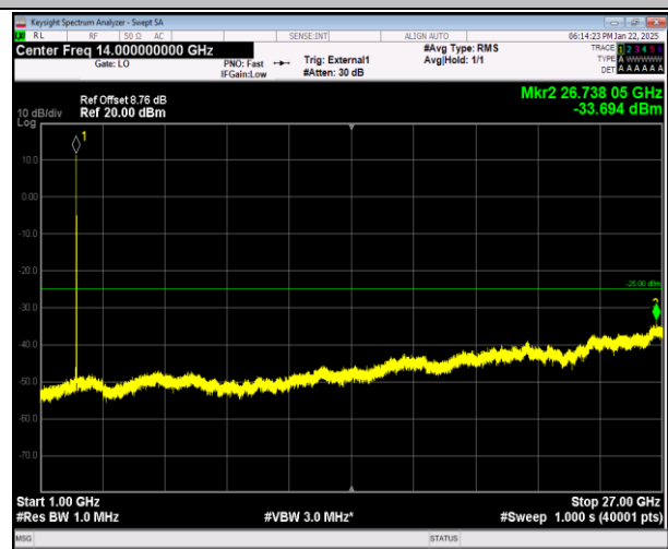
41-41-5MHz-20MHz-QPSK-QPSK-39683-39800-1RB#0-1RB#99-1000~27000MHz-PASS
