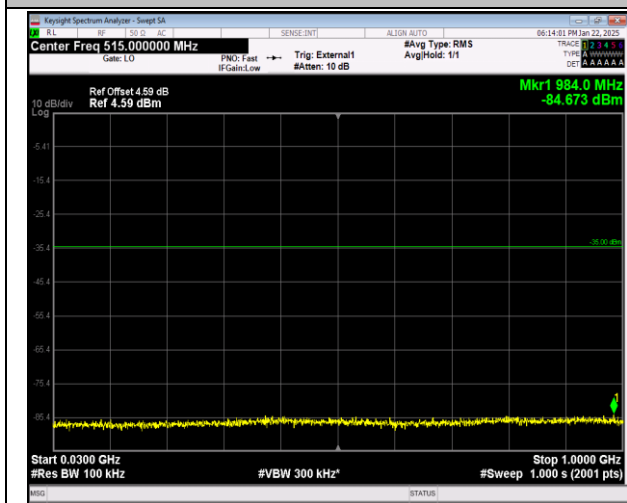
41-41-5MHz-20MHz-QPSK-QPSK-39683-39800-1RB#0-1RB#99-30~1000MHz-PASS
