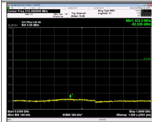
41-41-5MHz-20MHz-QPSK-QPSK-40528-40645-1RB#24-0-0RB#0-30~1000MHz-PASS
