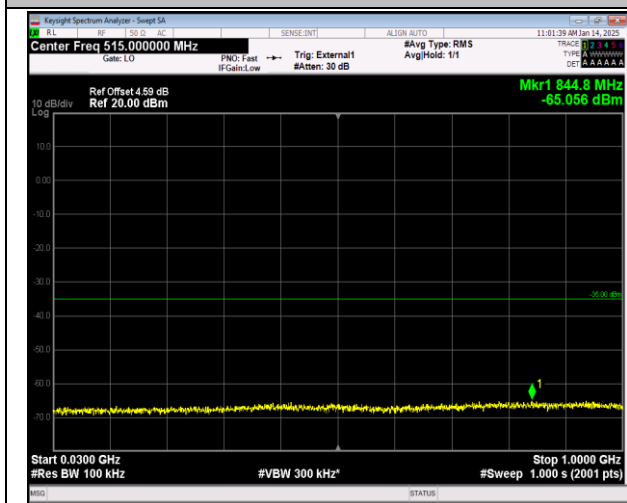
38-38-20MHz-20MHz-QPSK-QPSK-37952-38150-1RB#0 -0RB#0-30~1000MHz-PASS
