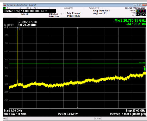
41-41-5MHz-20MHz-QPSK-QPSK-40528-40645-1RB#24-0-0RB#0-1000~27000MHz-PASS
