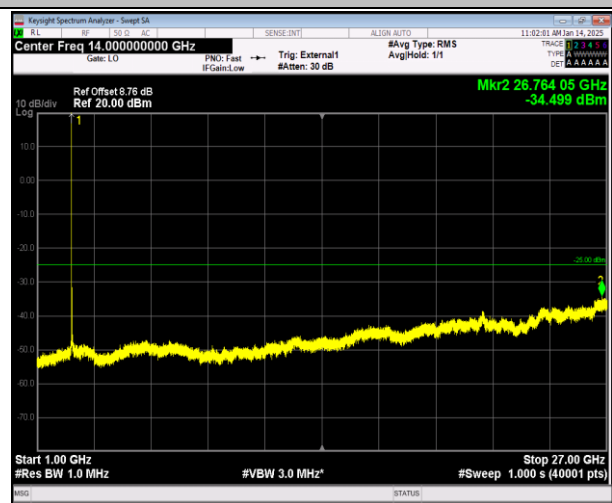
38-38-20MHz-20MHz-QPSK-QPSK-37952-38150-1RB#0-0 RB#0-1000~27000MHz-PASS
