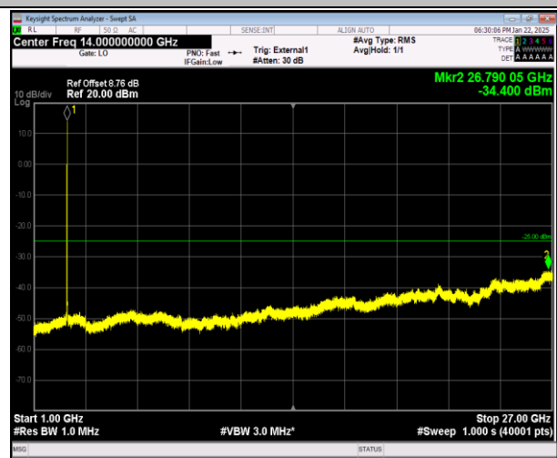
41-41-5MHz-20MHz-QPSK-QPSK-41373-41490-25RB#0-1 00RB#0-1000~27000MHz-PASS
