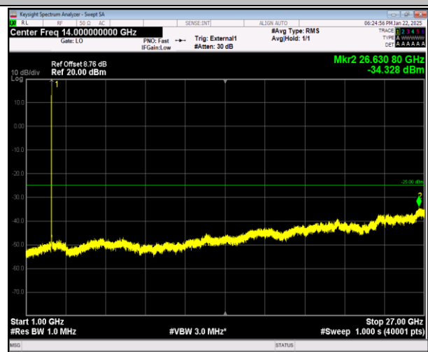
41-41-5MHz-20MHz-QPSK-QPSK-41373-41490-1RB#0-0RB#0-1000~27000MHz-PASS
