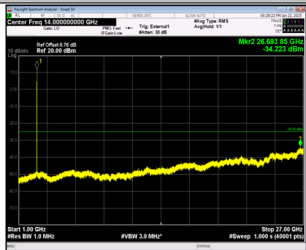
41-41-5MHz-20MHz-QPSK-QPSK-41373-41490-1RB#0-0RB#99-1000~27000MHz-PASS
