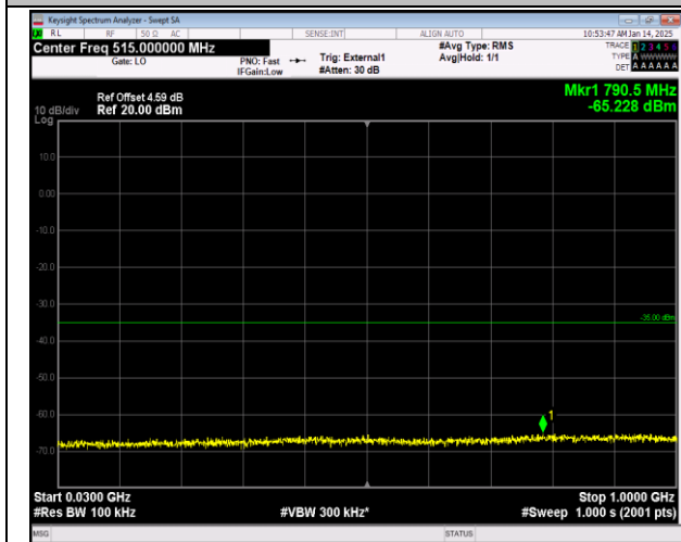
38-38-20MHz-20MHz-QPSK-QPSK-37901-38099-1RB#0 -0RB#0-30~1000MHz-PASS
