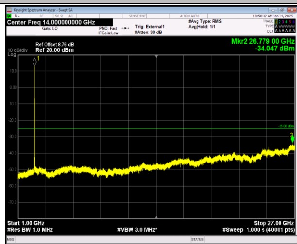
38-38-20MHz-20MHz-QPSK-QPSK-37850-38048-1RB#0-1 RB#99-1000~27000MHz-PASS
