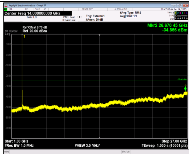
38-38-20MHz-20MHz-QPSK-QPSK-37850-38048-1RB#0-0 RB#0-1000~27000MHz-PASS
