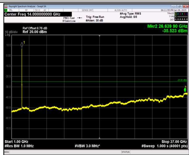
7-7-20MHz-20MHz-QPSK-QPSK-21152-21350-100RB#0-1 00RB#0-1000~27000MHz-PASS
