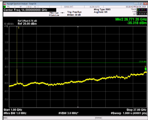
7-7-10MHz-20MHz-QPSK-QPSK-20805-20949-1RB#0-ORB #0-1000~27000MHz-PASS
