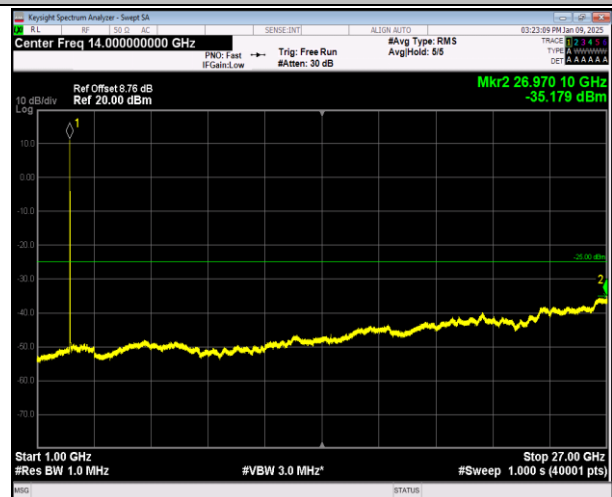
7-7-10MHz-20MHz-QPSK-QPSK-20805-20949-1RB#0-1RB #99-1000~27000MHz-PASS
