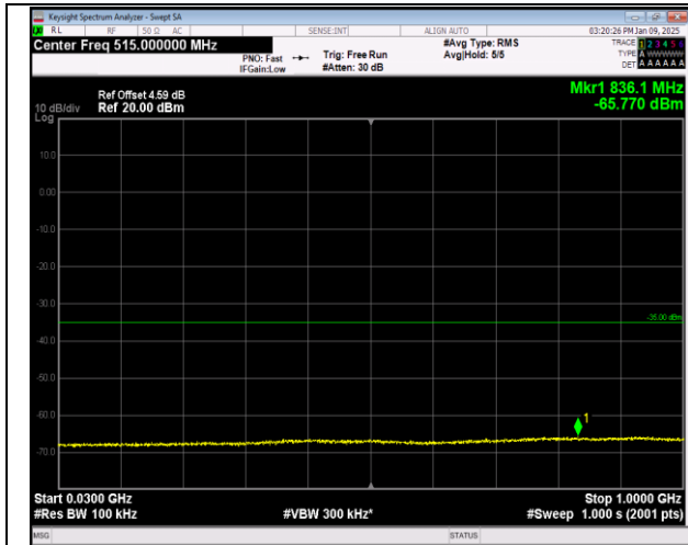
7-7-10MHz-20MHz-QPSK-QPSK-20805-20949-1RB#0-0 RB#0-30~1000MHz-PASS
