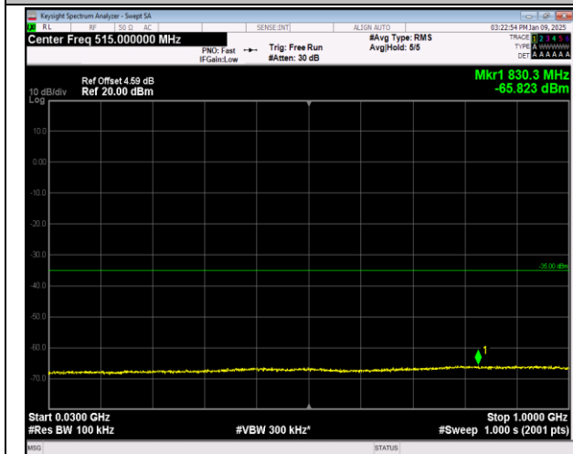
7-7-10MHz-20MHz-QPSK-QPSK-20805-20949-1RB#0-1 RB#99-30~1000MHz-PASS
