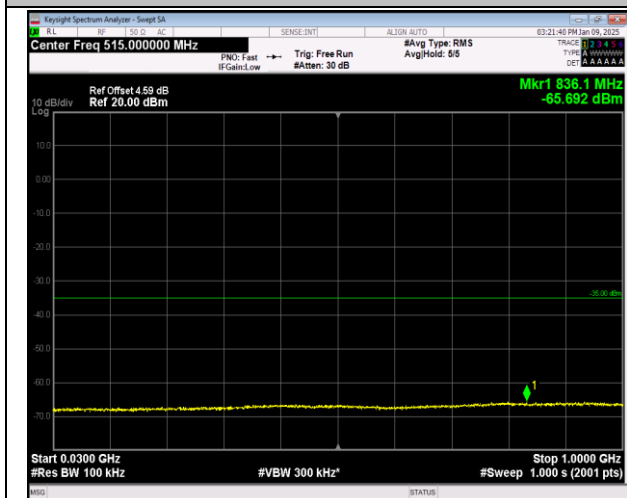
7-7-10MHz-20MHz-QPSK-QPSK-20805-20949-1RB#49-
