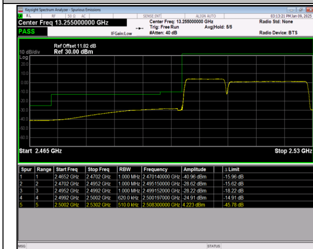
7-7-10MHz-20MHz-QPSK@QPSK-QPSK@QPSK-20805-
