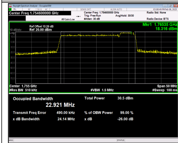
66-66-20MHz-5MHz-QPSK-QPSK-132397-132514-100R B#0-25RB#0-PASS
