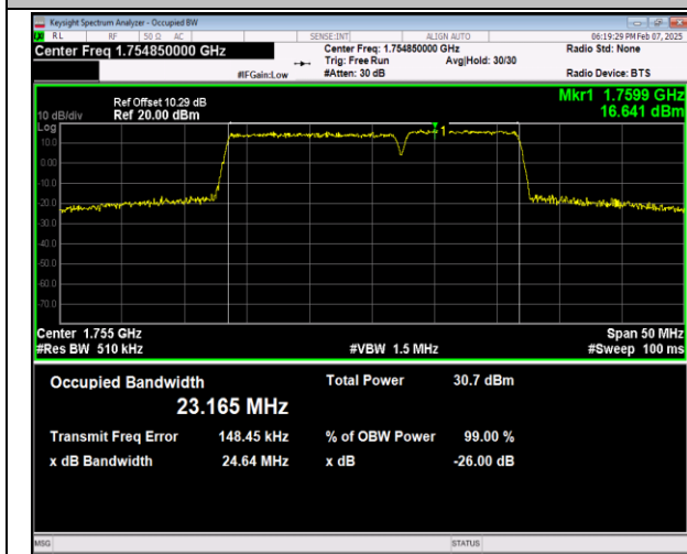
66-66-15MHz-10MHz-QPSK-QPSK-132373-132493-75R B#0-50RB#0-PASS
