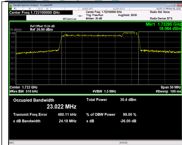
66-66-20MHz-5MHz-QPSK-QPSK-132072-132189-100R B#0-25RB#0-PASS
