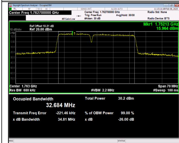
66-66-15MHz-20MHz-QPSK-QPSK-132401-132572-75R B#0-100RB#0-PASS
