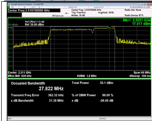
41-41-20MHz-10MHz-QPSK-QPSK-39750-39894-100RB #0-50RB#0-PASS
