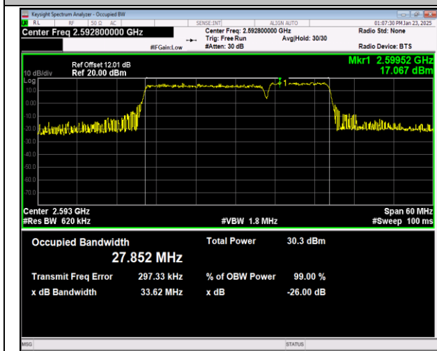
41-41-20MHz-10MHz-QPSK-QPSK-40571-40715-100RB #0-50RB#0-PASS
