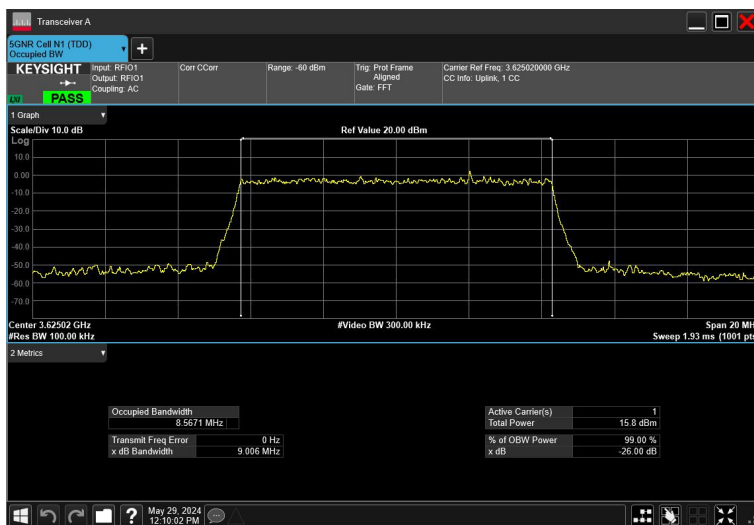
10MHz_30kHz_3625MHz_CP-OFDM 256QAM_RB24@0
