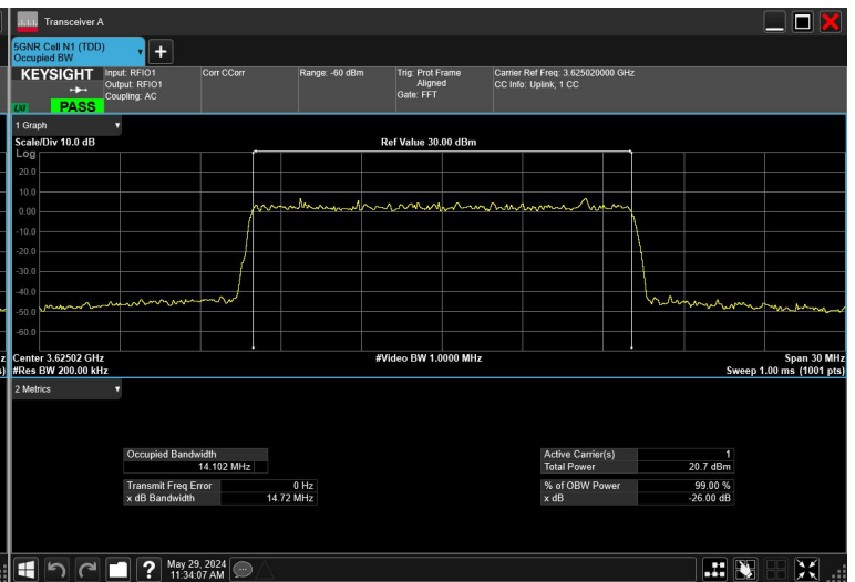
15MHz_15kHz_3625MHz_CP-OFDM QPSK_RB79@0
