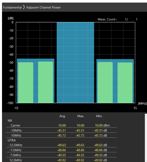
10MHz_30kHz_3695MHz_DFT-s-OFDM QPSK_RB24@0 -45.31 dB,-45.72 dB
