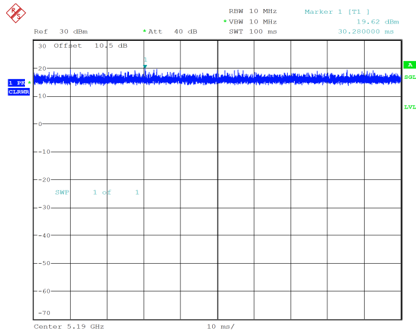
n40_5190MHz_Chain 0 100.000 ms
