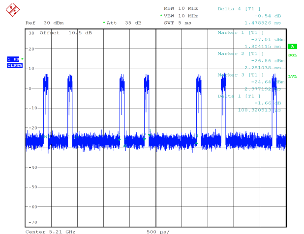
ax80_5210MHz_RU_484/65_Chain 0
