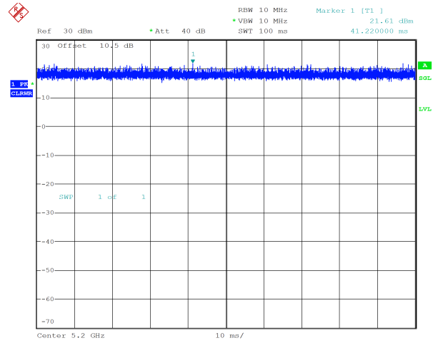
n20_5200MHz_Chain 0 100.000 ms
