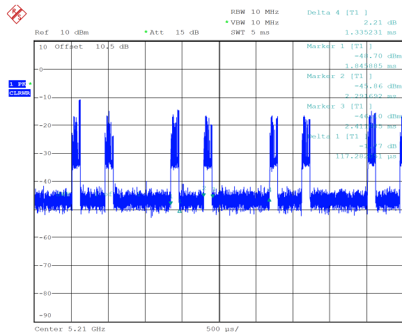
ax80_5210MHz_RU_242/61_Chain 0
