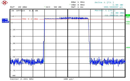
\pi/4 -DQPSK_Hopping_2DH1 0.407ms
