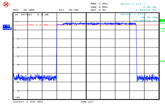
8DPSK_Hopping_3DH3 1.666ms
