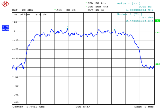
\pi/4 -DQPSK_Middle 1.004MHz
