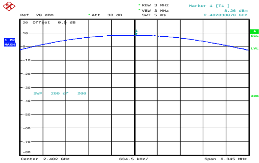
\pi/4 -DQPSK_Low 8.26dBm
