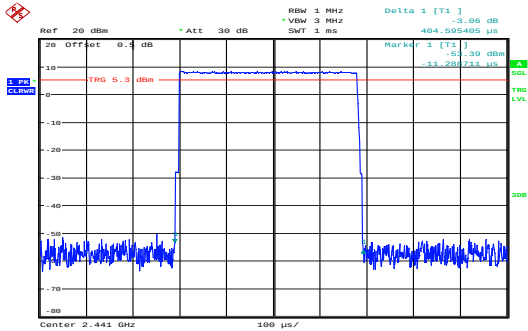
GFSK_Hopping_DH1 0.405ms
