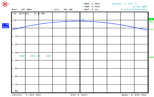
\pi/4 -DQPSK_Middle 8.53dBm
