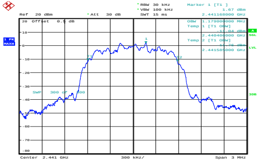
\pi/4 -DQPSK_Middle 1.179MHz
