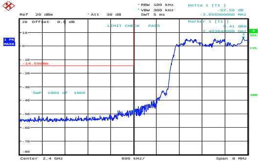
\pi/4 -DQPSK_Hopping_Lower
