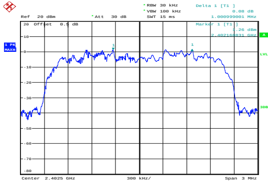
\pi/4 -DQPSK_Low 1.001MHz
