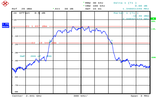
\pi/4 -DQPSK_Middle 1.349MHz
