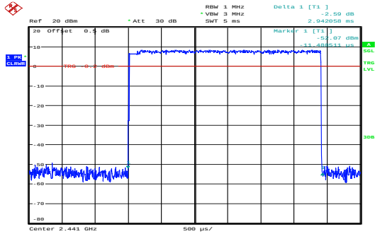
\pi/4 -DQPSK_Hopping_2DH5 2.942ms
