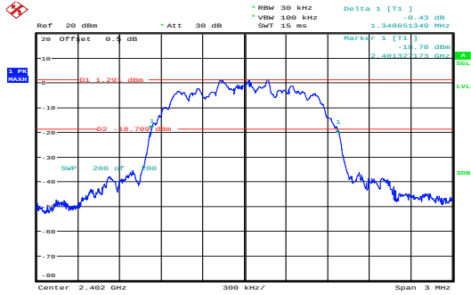
\pi/4 -DQPSK_Low 1.349MHz
