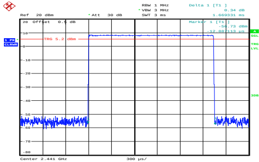
GFSK_Hopping_DH3 1.669ms
