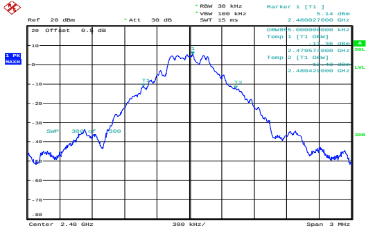
GFSK_High 0.855MHz
