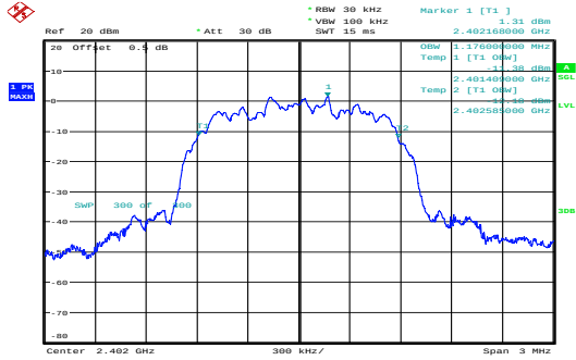
\pi/4 -DQPSK_Low 1.176MHz
