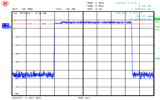
\pi/4 -DQPSK_Hopping_2DH3 1.669ms
