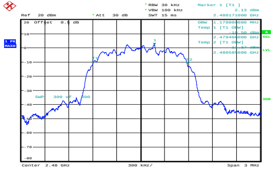
\pi/4 -DQPSK_High 1.179MHz
