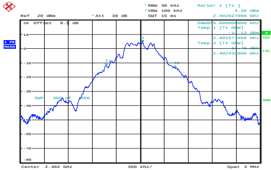
GFSK_Low 0.858MHz
