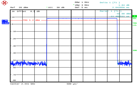
GFSK_Hopping_DH5 2.942ms
