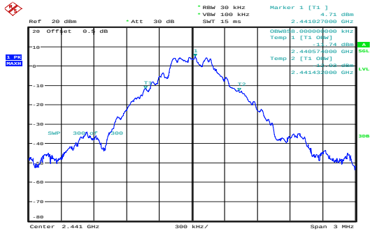
GFSK_Middle 0.858MHz
