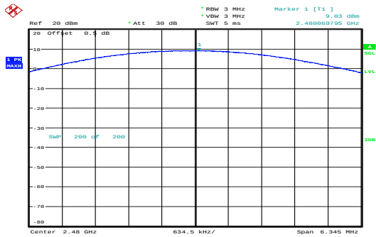
\pi/4 -DQPSK_High 9.03dBm
