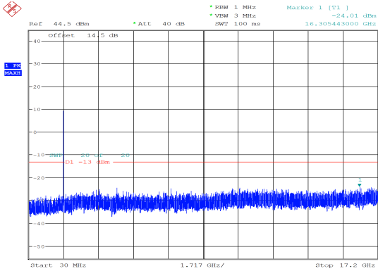
20MHz_Low_QPSK_100@0 -24.01 dBm
