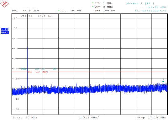
10MHz_Low_QPSK_50@0 -23.63 dBm
