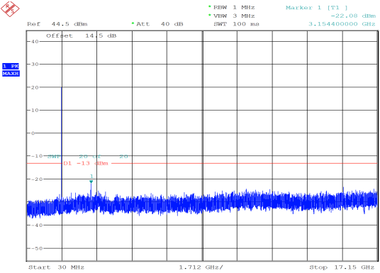
10MHz_Low_QPSK_1@0 -22.08 dBm
