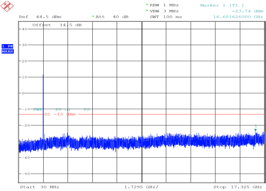
10MHz_Middle_QPSK_50@0 -23.74 dBm
