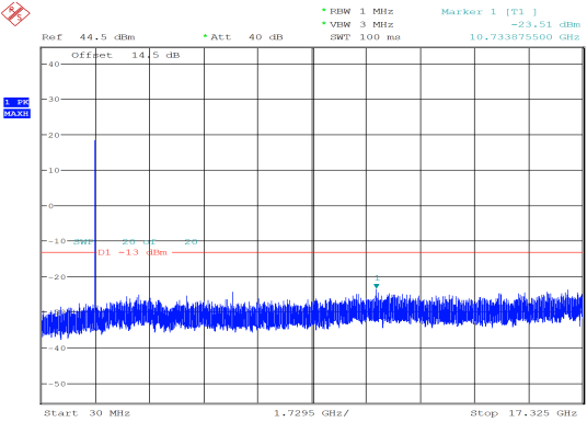
10MHz_Middle_QPSK_1@0 -23.51 dBm
