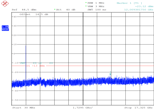
20MHz_Middle_QPSK_100@0 -23.12 dBm
