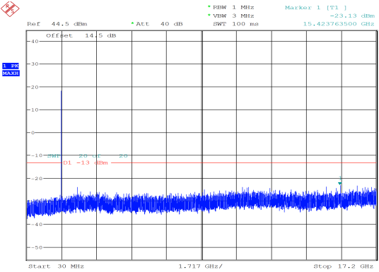
20MHz_Low_QPSK_1@0 -23.13 dBm
