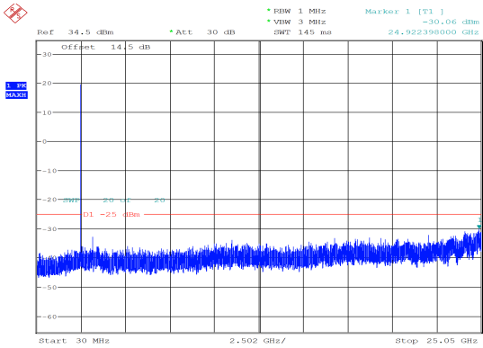
10MHz_Low_QPSK_1@0 -30.06 dBm
