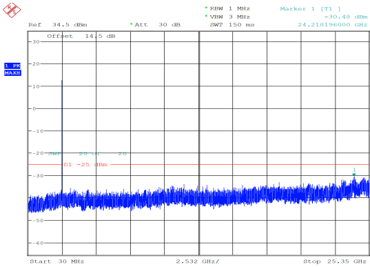
10MHz_Middle_QPSK_50@0 -30.48 dBm
