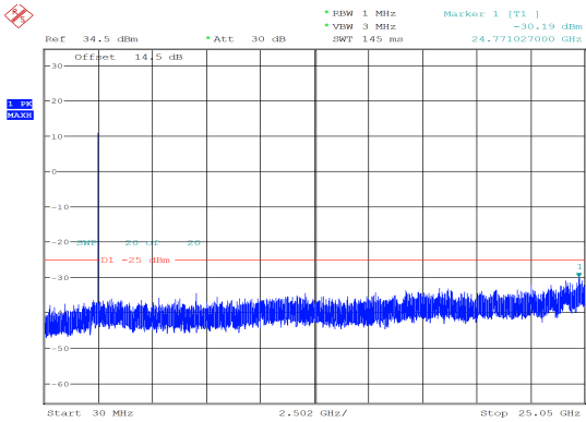
10MHz_Low_QPSK_50@0 -30.19 dBm
