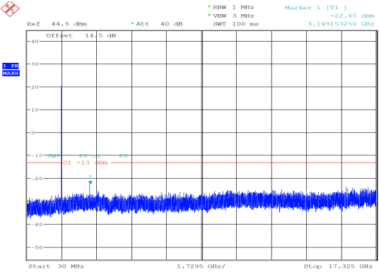
20MHz_Middle_QPSK_1@0 -22.65 dBm
