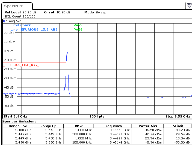
100MHz_30kHz_3500MHz_DFT-s-OFDM QPSK_RB1@0 -23.34 dBm
