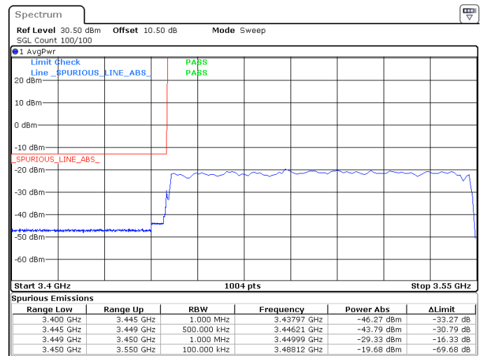
100MHz_30kHz_3500MHz_DFT-s-OFDM QPSK_RB270@0 -29.33 dBm
