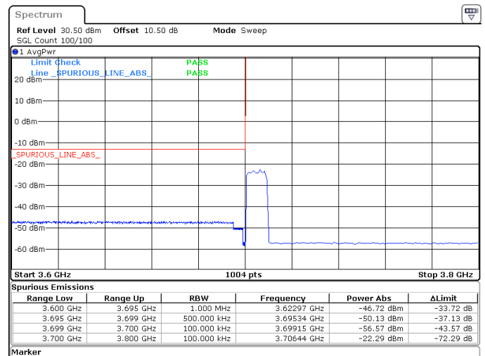
10MHz_15kHz_3705MHz_DFT-s-OFDM QPSK_RB50@0 -46.72 dBm
