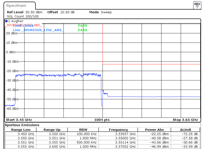
90MHz_30kHz_3505MHz_DFT-s-OFDM QPSK_RB243@0 -40.58 dBm
