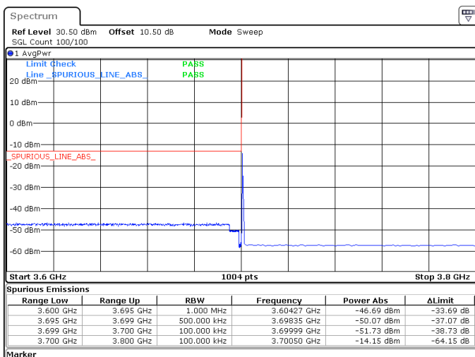
10MHz_15kHz_3705MHz_DFT-s-OFDM QPSK_RB1@0 -46.69 dBm
