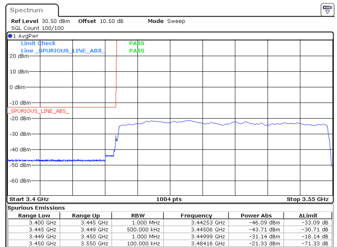
100MHz_30kHz_3500MHz_DFT-s-OFDM QPSK_RB270@0 -31.14 dBm
