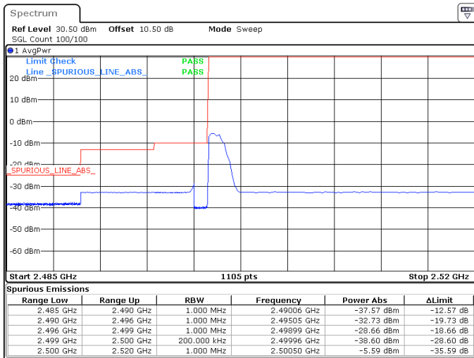
20MHz_15kHz_2510MHz_DFT-s-OFDM QPSK_RB1@0 -37.57 dBm
