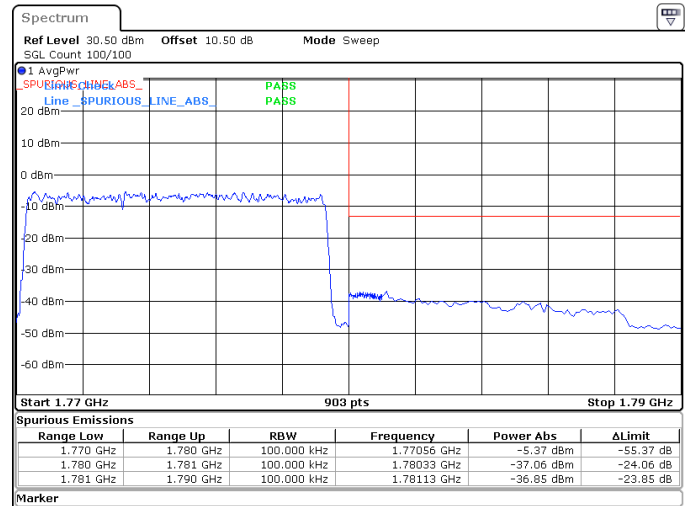
10MHz_15kHz_1775MHz_DFT-s-OFDM QPSK_RB50@0 -36.85 dBm
