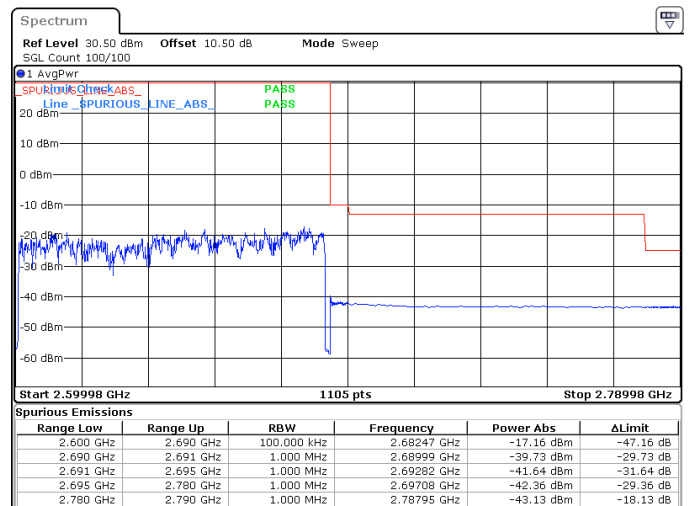
90MHz_30kHz_2644.98MHz_DFT-s-OFDM QPSK_RB243@0 -43.13 dBm
