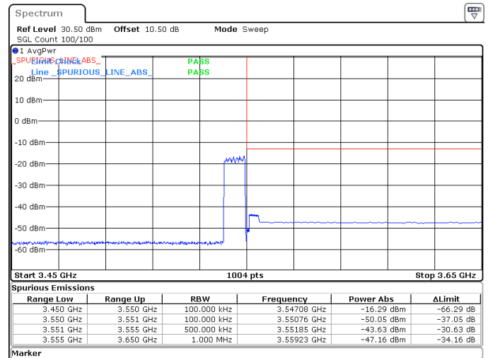
10MHz_15kHz_3545MHz_DFT-s-OFDM QPSK_RB50@0 -43.63 dBm
