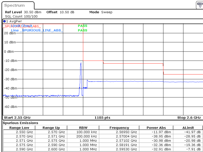
20MHz_15kHz_2560MHz_DFT-s-OFDM QPSK_RB1@105 -32.91 dBm
