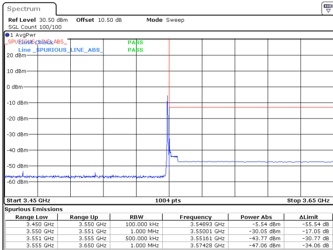
90MHz_30kHz_3505MHz_DFT-s-OFDM QPSK_RB1@244 -30.05 dBm
