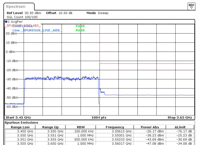
80MHz_30kHz_3510MHz_DFT-s-OFDM QPSK_RB216@0 -38.23 dBm
