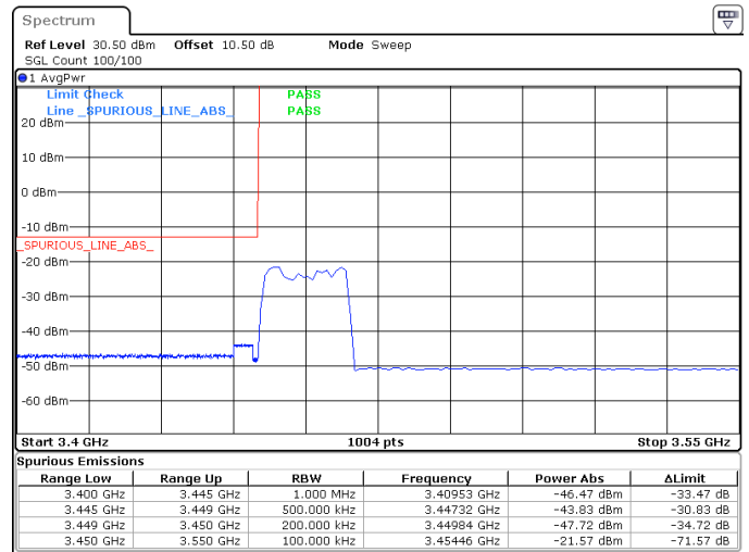
20MHz_30kHz_3460MHz_DFT-s-OFDM QPSK_RB50@0 -43.83 dBm
