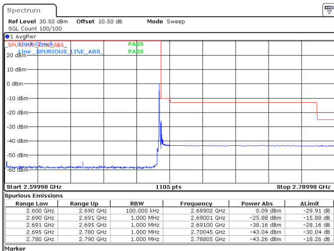
90MHz_30kHz_2644.98MHz_DFT-s-OFDM QPSK_RB1@244 -25.88 dBm
