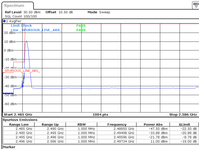
90MHz_30kHz_2541MHz_DFT-s-OFDM QPSK_RB1@0 -21.78 dBm
