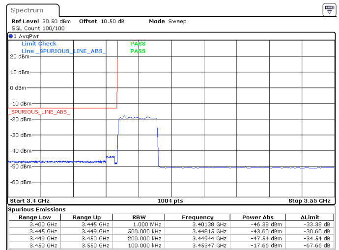
20MHz_15kHz_3460MHz_DFT-s-OFDM QPSK_RB100@0 -43.60 dBm
