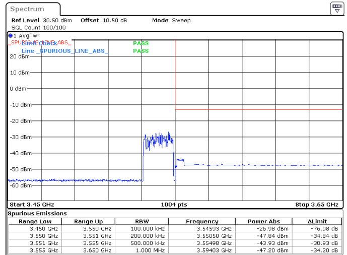
20MHz_30kHz_3540MHz_DFT-s-OFDM QPSK_RB50@0 -43.93 dBm
