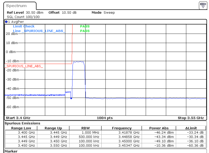
10MHz_15kHz_3455MHz_DFT-s-OFDM QPSK_RB50@0 -43.34 dBm
