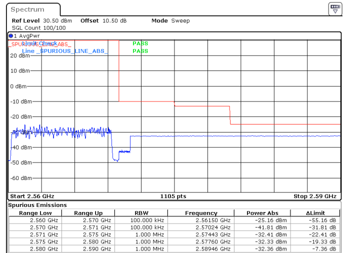
10MHz_15kHz_2565MHz_DFT-s-OFDM QPSK_RB50@0 -32.36 dBm
