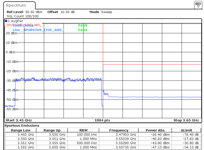
90MHz_30kHz_3505MHz_DFT-s-OFDM QPSK_RB243@0 -40.83 dBm
