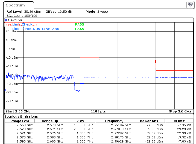
20MHz_15kHz_2560MHz_DFT-s-OFDM QPSK_RB100@0 -32.83 dBm
