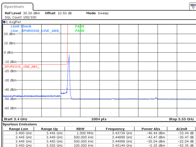
70MHz_30kHz_3485MHz_DFT-s-OFDM QPSK_RB1@0 -35.04 dBm
