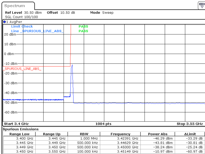
60MHz_30kHz_3480MHz_DFT-s-OFDM QPSK_RB1@0 -38.24 dBm
