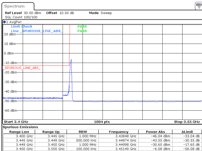
100MHz_30kHz_3500MHz_DFT-s-OFDM QPSK_RB1@0 -30.65 dBm
