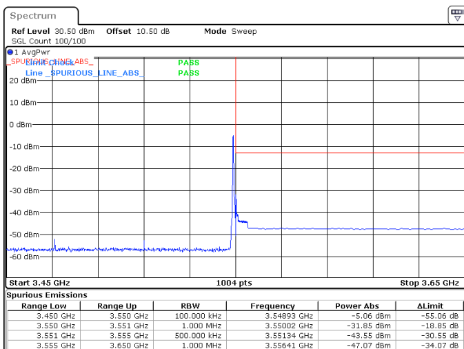
80MHz_30kHz_3510MHz_DFT-s-OFDM QPSK_RB1@216 -31.85 dBm
