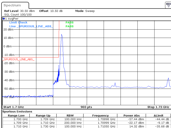
20MHz_15kHz_1720MHz_DFT-s-OFDM QPSK_RB1@0 -22.17 dBm
