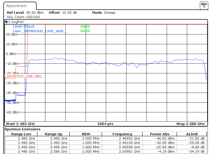
90MHz_30kHz_2541MHz_DFT-s-OFDM QPSK_RB243@0 -22.68 dBm
