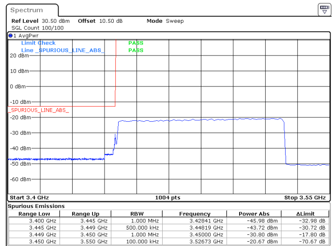
80MHz_30kHz_3490MHz_DFT-s-OFDM QPSK_RB216@0 -30.80 dBm
