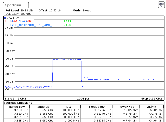
40MHz_30kHz_3530MHz_DFT-s-OFDM QPSK_RB100@0 -43.76 dBm
