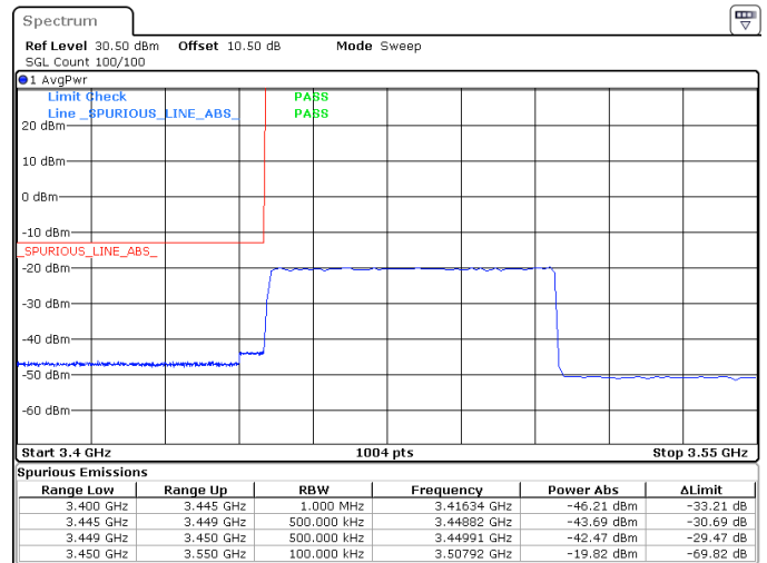
60MHz_30kHz_3480MHz_DFT-s-OFDM QPSK_RB162@0 -42.47 dBm
