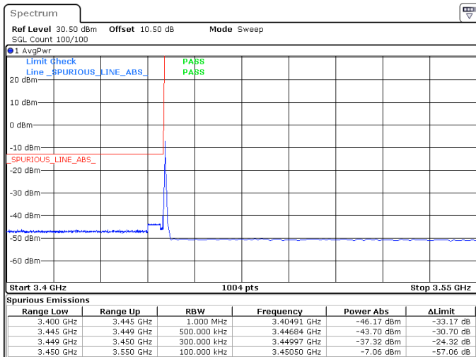
30MHz_15kHz_3465MHz_DFT-s-OFDM QPSK_RB1@0 -37.32 dBm
