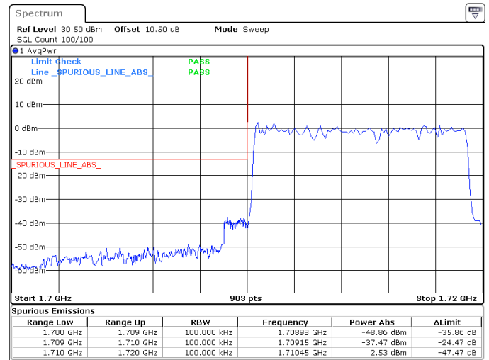
10MHz_15kHz_1715MHz_DFT-s-OFDM QPSK_RB50@0 -37.47 dBm
