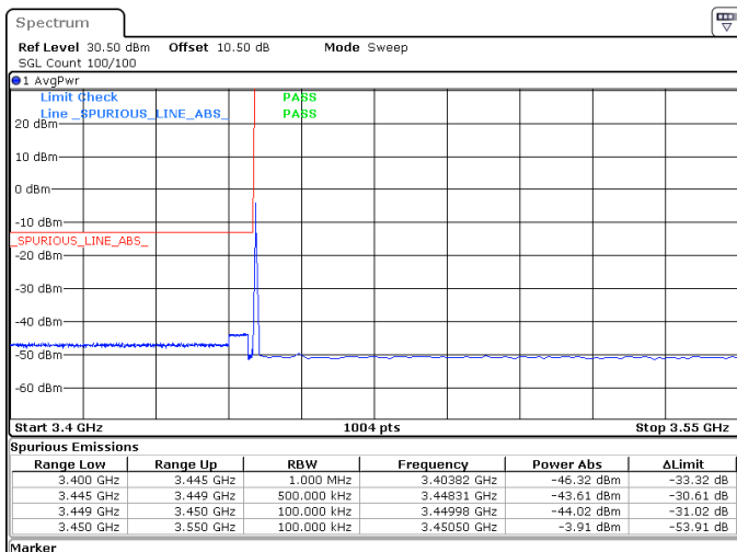
10MHz_15kHz_3455MHz_DFT-s-OFDM QPSK_RB1@0 -43.61 dBm
