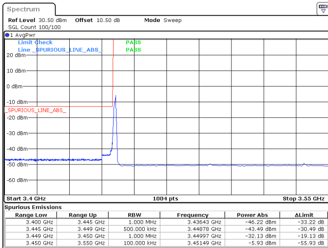
90MHz_30kHz_3495MHz_DFT-s-OFDM QPSK_RB1@0 -32.13 dBm
