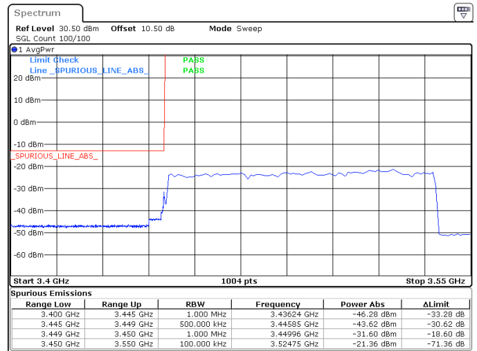
90MHz_30kHz_3495MHz_DFT-s-OFDM QPSK_RB243@0 -31.60 dBm
