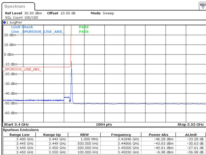
20MHz_15kHz_3460MHz_DFT-s-OFDM QPSK_RB1@0 -40.61 dBm
