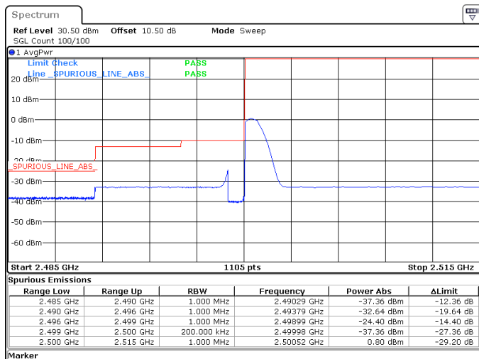
15MHz_15kHz_2507.5MHz_DFT-s-OFDM QPSK_RB1@0 -37.36 dBm
