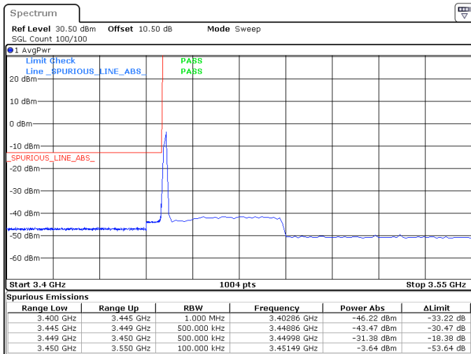
40MHz_30kHz_3470MHz_DFT-s-OFDM QPSK_RB1@0 -31.38 dBm
