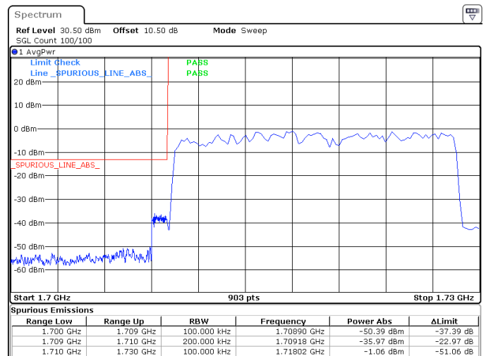
20MHz_15kHz_1720MHz_DFT-s-OFDM QPSK_RB100@0 -35.97 dBm
