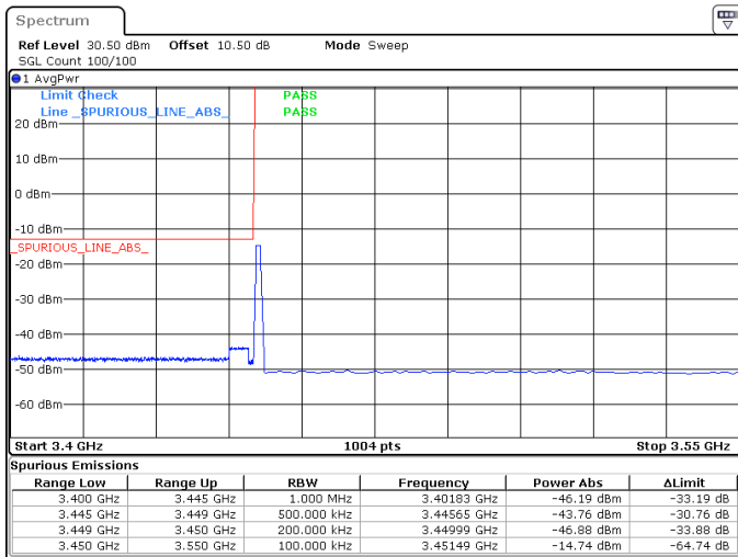
20MHz_30kHz_3460MHz_DFT-s-OFDM QPSK_RB1@0 -43.76 dBm
