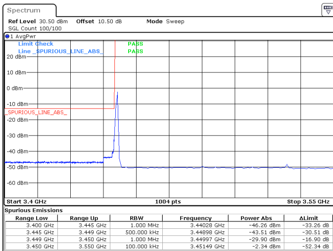
80MHz_30kHz_3490MHz_DFT-s-OFDM QPSK_RB1@0 -29.90 dBm
