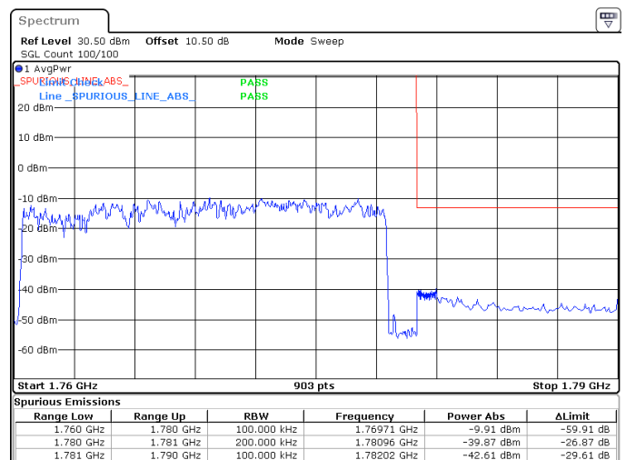
20MHz_15kHz_1770MHz_DFT-s-OFDM QPSK_RB100@0 -39.87 dBm
