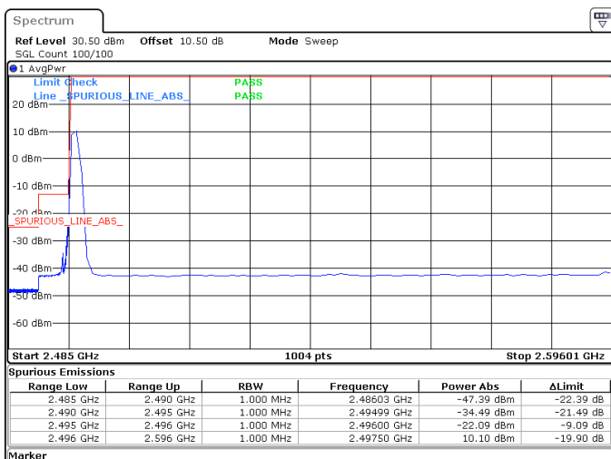
100MHz_30kHz_2546.01MHz_DFT-s-OFDM QPSK_RB1@0 -22.09 dBm
