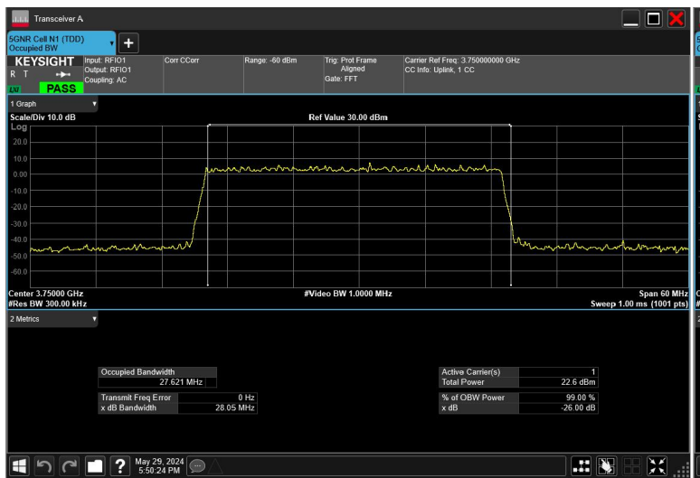
30MHz_30kHz_3750MHz_DFT-s-OFDM \pi/2 BPSK_RB75@0
