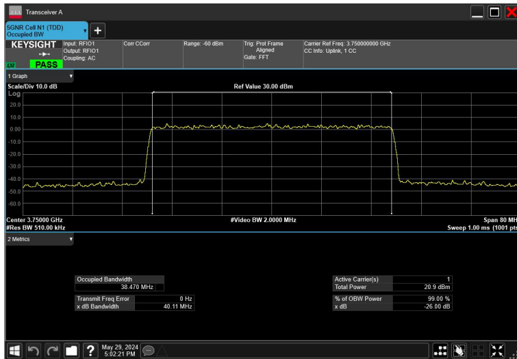
40MHz_15kHz_3750MHz_CP-OFDM QPSK_RB216@0
