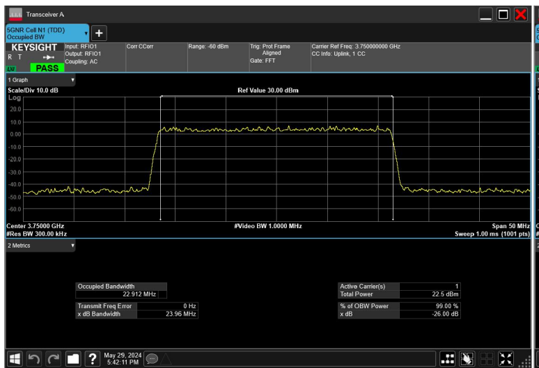
25MHz_30kHz_3750MHz_DFT-s-OFDM \pi/2 BPSK_RB64@0
