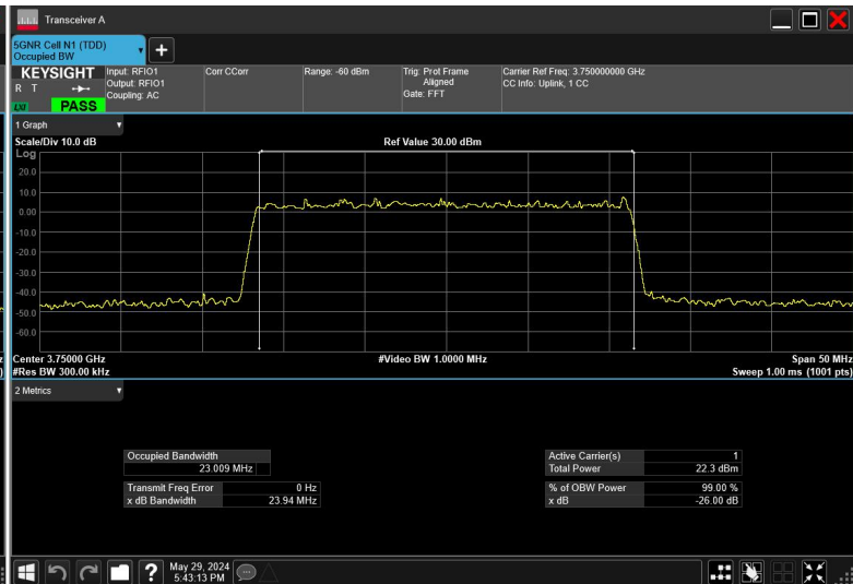
25MHz_30kHz_3750MHz_DFT-s-OFDM QPSK_RB64@0
