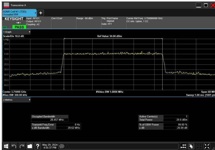
30MHz_15kHz_3750MHz_CP-OFDM QPSK_RB160@0
