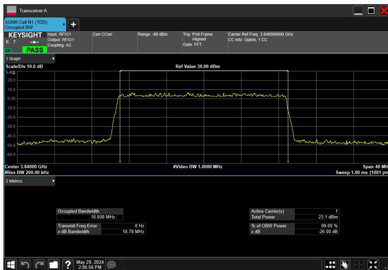
20MHz_30kHz_3840MHz_DFT-s-OFDM \pi/2 BPSK_RB50@0
