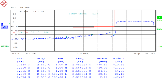
10MHz_Low_QPSK_50@0
