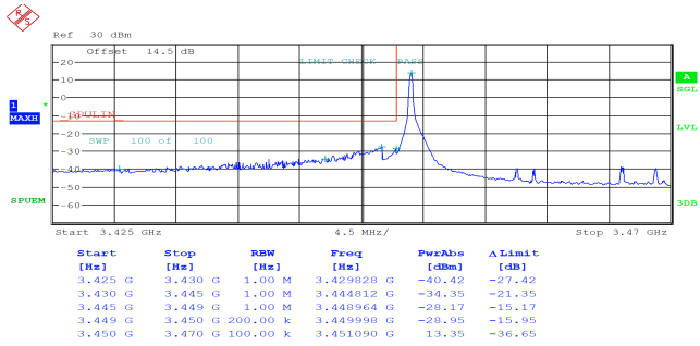
20MHz_Low_QPSK_1@0
