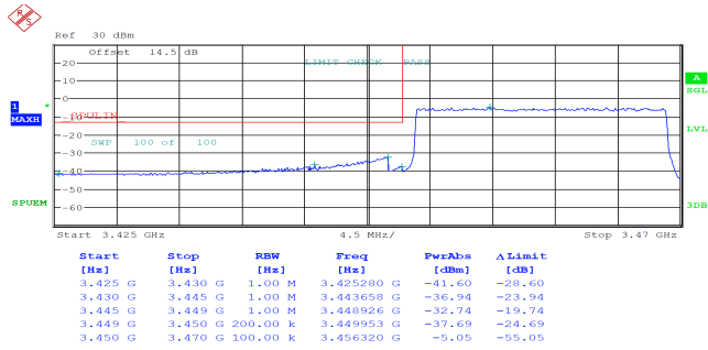
20MHz_Low_QPSK_100@0
