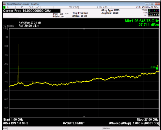
Band7_20MHz_QPSK_21350_1RB#0_1000~27000_1000~27000
