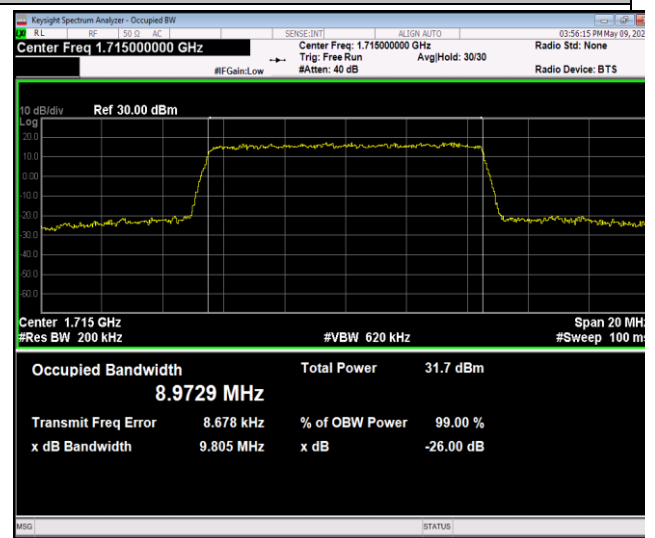
Band4-10MHz-QPSK-20000-50RB#0-PASS
