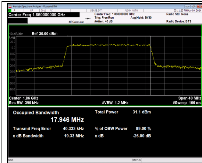
Band2-20MHz-16QAM-18700-100RB#0-PASS
