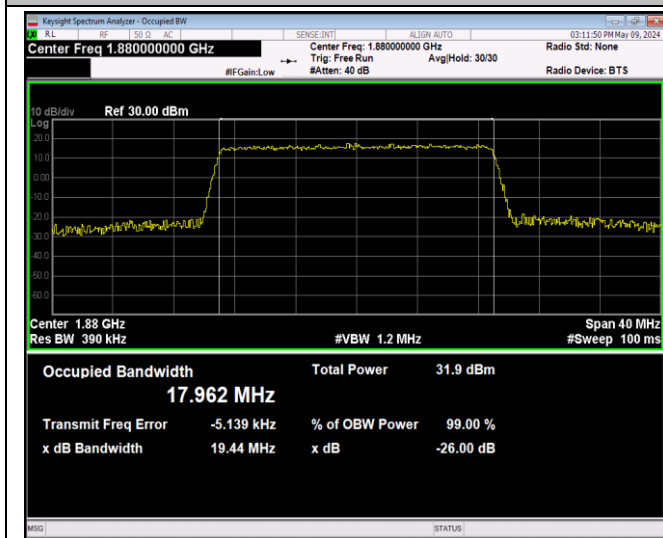
Band2-20MHz-QPSK-18900-100RB#0-PASS
