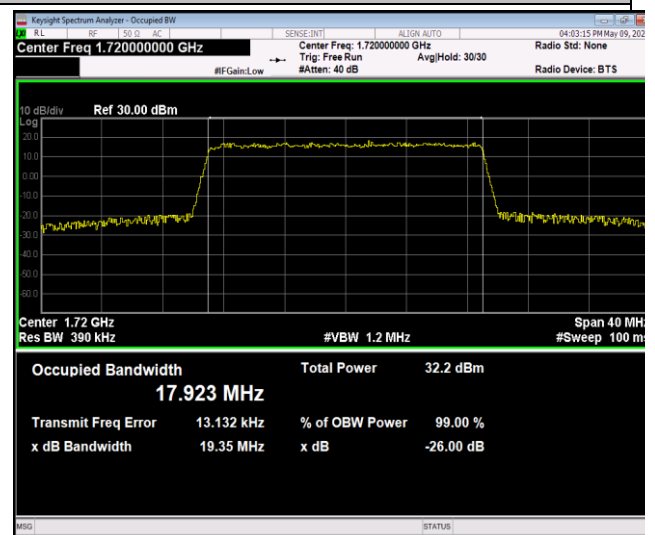
Band4-20MHz-QPSK-20050-100RB#0-PASS
