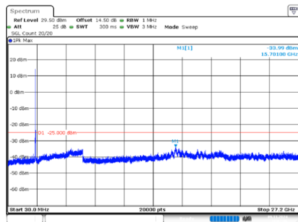
15MHz_Low_QPSK_75@0(30MHz~27.2GHz)
