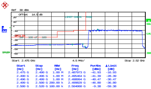
20MHz_Low_QPSK_100@0
