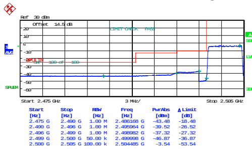
5MHz_Low_QPSK_25@0
