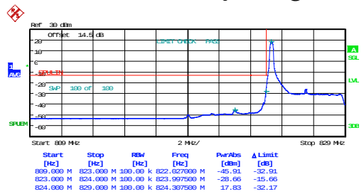
5MHz_Low_QPSK_1@0
