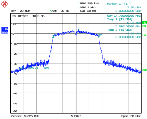
802.11n20_5825MHz 17.700MHz
