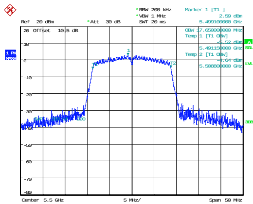
802.11n20_5500MHz 17.650MHz
