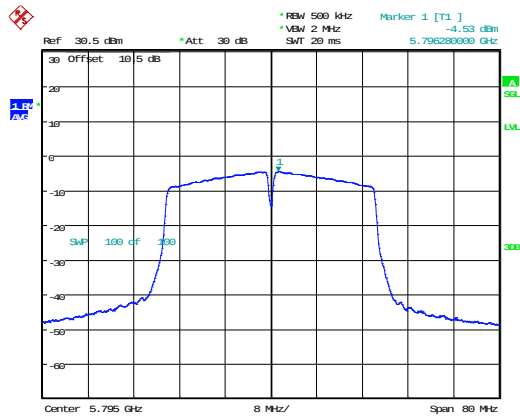
802.11n40_5795MHz
