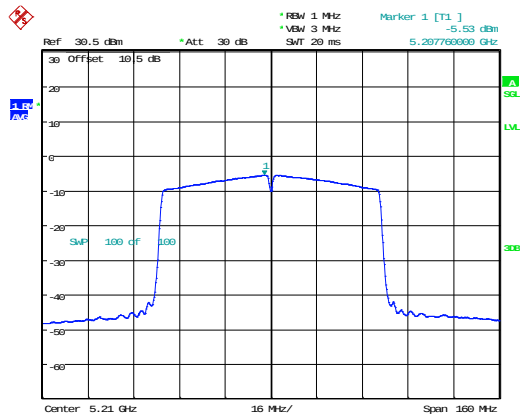
802.11ac80_5210MHz
