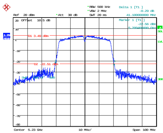
802.11n40_5230MHz 41.100MHz
