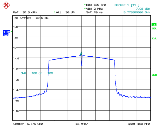
802.11ac80_5775MHz
