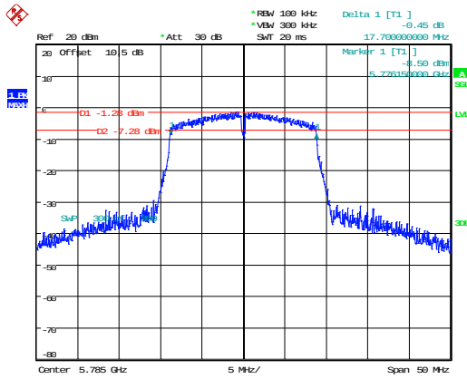
802.11n20_5785MHz 17.700MHz
