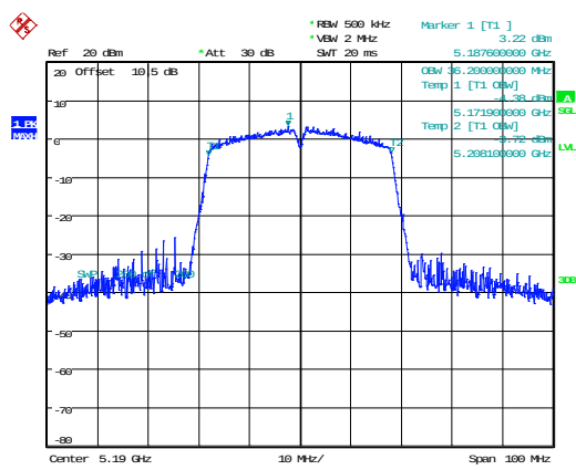
802.11n40_5190MHz 36.200MHz
