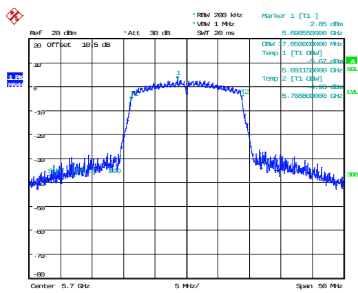
802.11n20_5700MHz 17.650MHz
