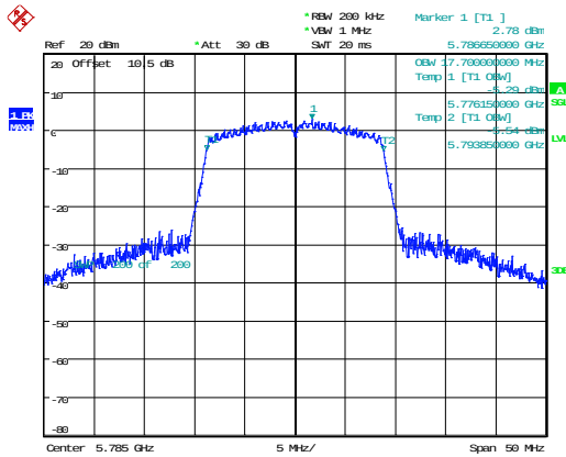
802.11n20_5785MHz 17.700MHz
