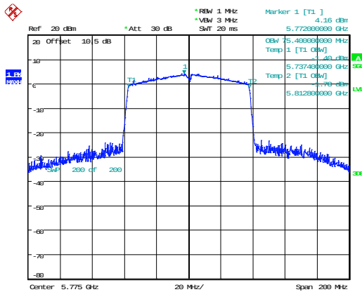
802.11ac80_5775MHz 75.400MHz
