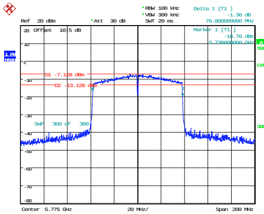
802.11ac80_5775MHz 76.800MHz
