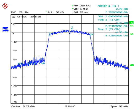
802.11n20_5720MHz 17.600MHz
