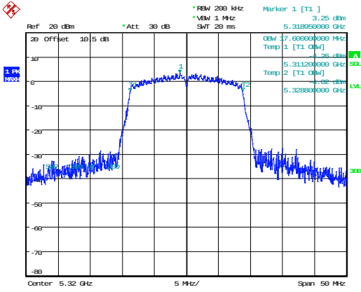
802.11n20_5320MHz 17.600MHz
