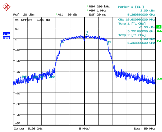
802.11a_5260MHz 16.600MHz
