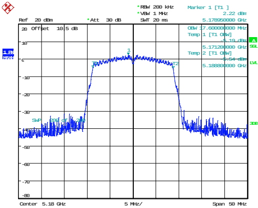
802.11n20_5180MHz 17.600MHz
