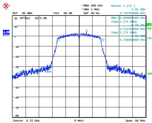
802.11a_5720MHz 16.600MHz
