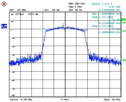
802.11n20_5280MHz 17.600MHz
