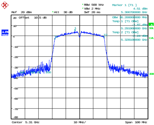
802.11n40_5310MHz 36.200MHz
