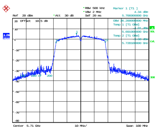
802.11n40_5710MHz 36.200MHz
