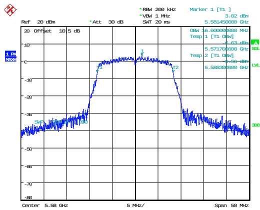
802.11a_5580MHz 16.600MHz
