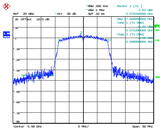
802.11n20_5580MHz 17.600MHz
