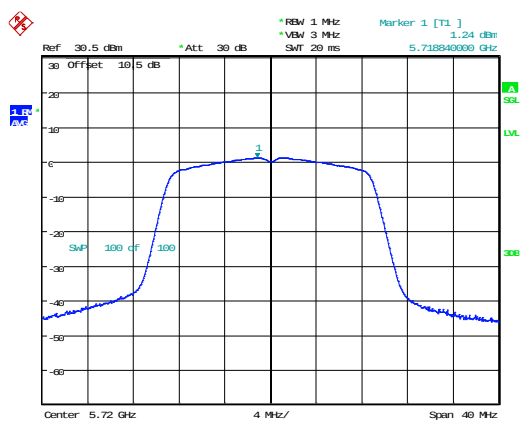
802.11n20_5720MHz
