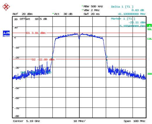
802.11n40_5190MHz 41.100MHz
