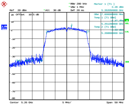
802.11n20_5260MHz 17.600MHz
