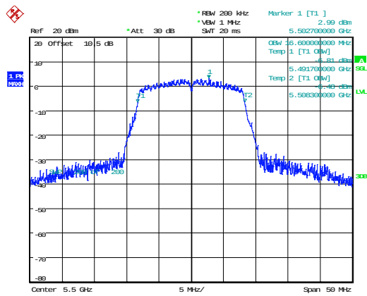
802.11a_5500MHz 16.600MHz
