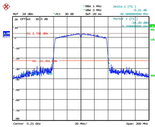
802.11ac80_5210MHz 82MHz
