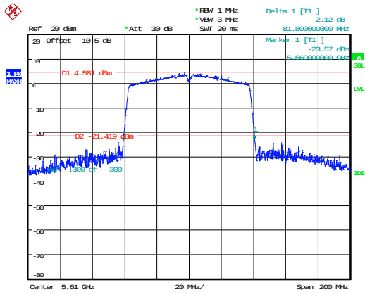
802.11ac80_5610MHz 81.800MHz
