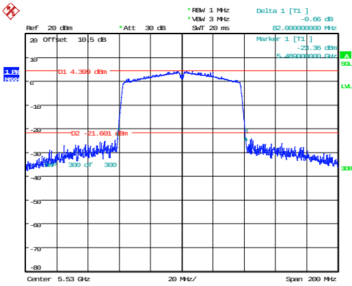
802.11ac80_5530MHz 82MHz
