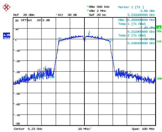
802.11n40_5230MHz 36.200MHz
