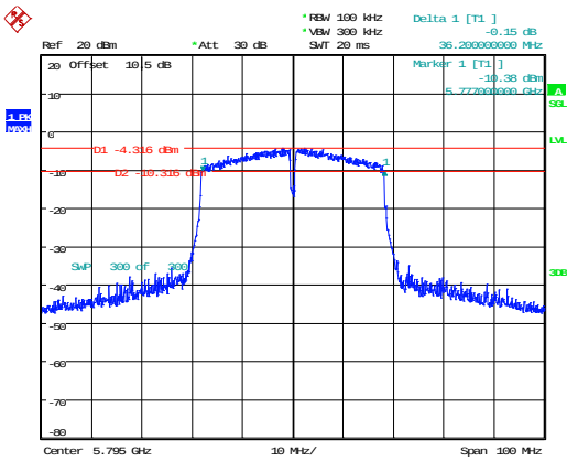
802.11n40_5795MHz 36.200MHz
