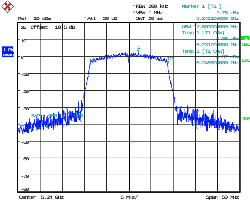
802.11n20_5240MHz 17.600MHz
