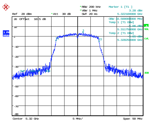
802.11a_5320MHz 16.500MHz
