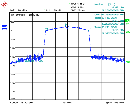
802.11ac80_5290MHz 75.200MHz
