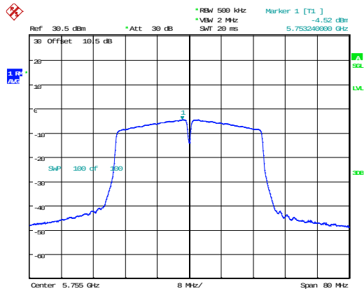
802.11n40_5755MHz
