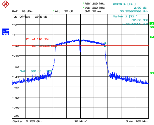
802.11n40_5755MHz 36.300MHz
