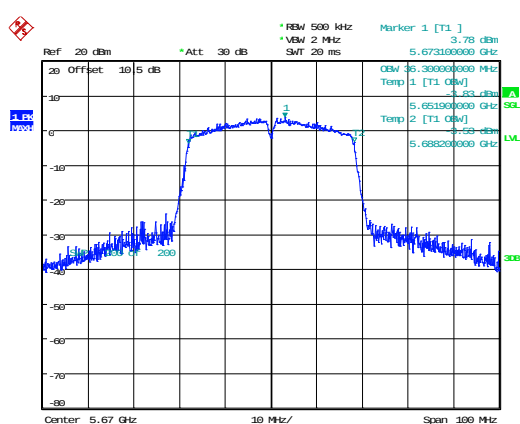
802.11n40_5670MHz 36.300MHz
