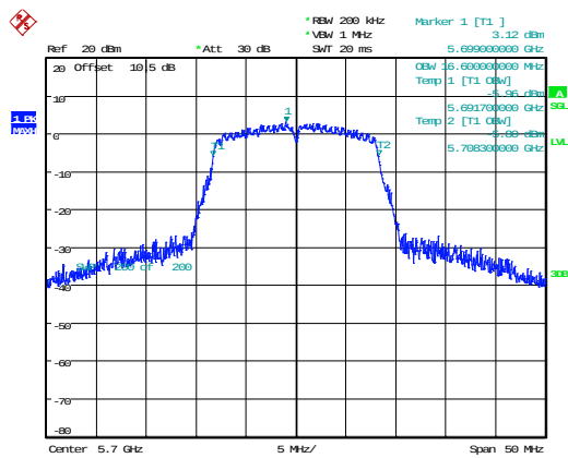
802.11a_5700MHz 16.600MHz
