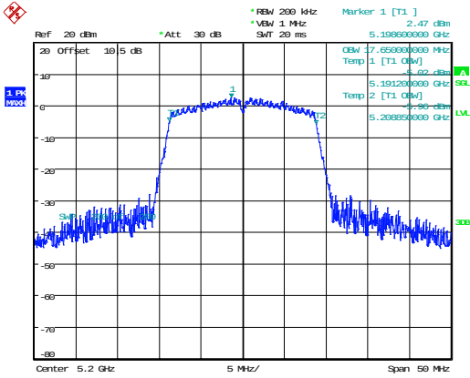
802.11n20_5200MHz 17.650MHz
