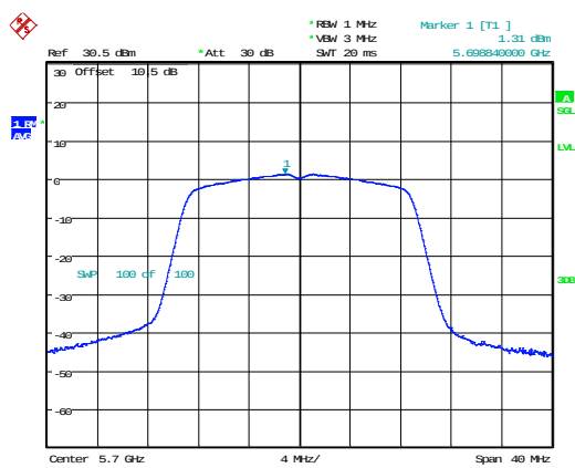
802.11n20_5700MHz
