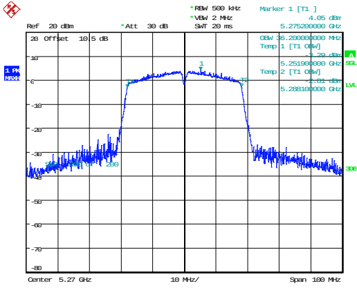
802.11n40_5270MHz 36.200MHz
