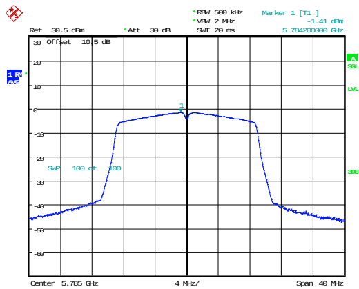
802.11n20_5785MHz
