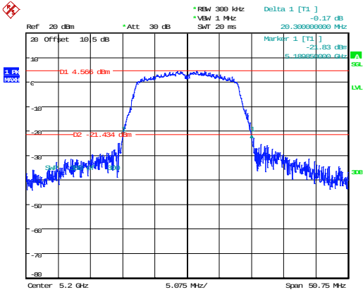
802.11a_5200MHz 20.300MHz
