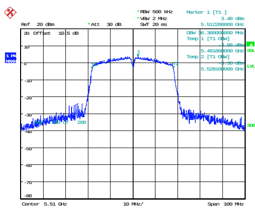
802.11n40_5510MHz 36.300MHz
