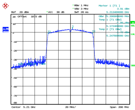
802.11ac80_5210MHz 75.200MHz
