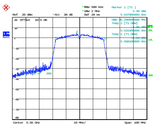
802.11n40_5550MHz 36.200MHz
