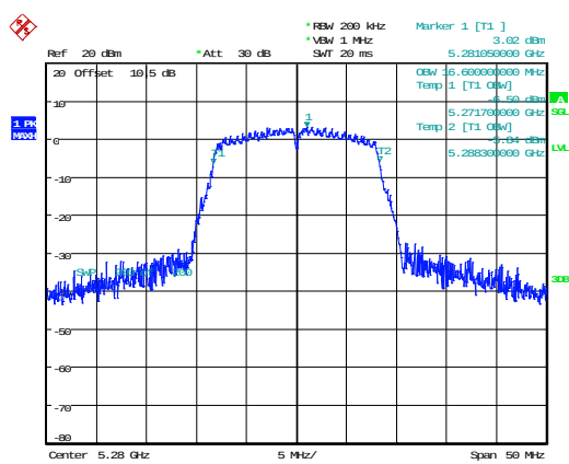
802.11a_5280MHz 16.600MHz
