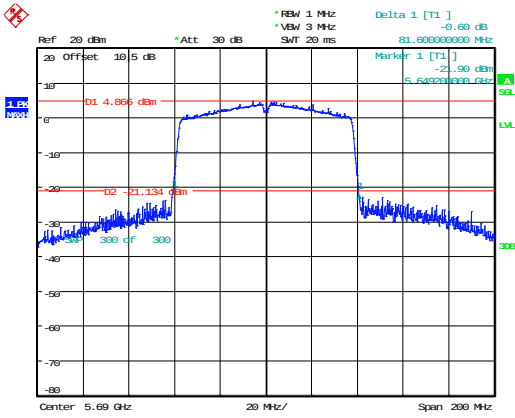
802.11ac80_5690MHz 81.600MHz
