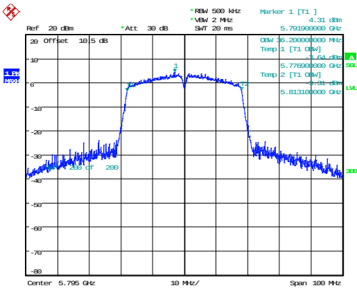
802.11n40_5795MHz 36.200MHz
