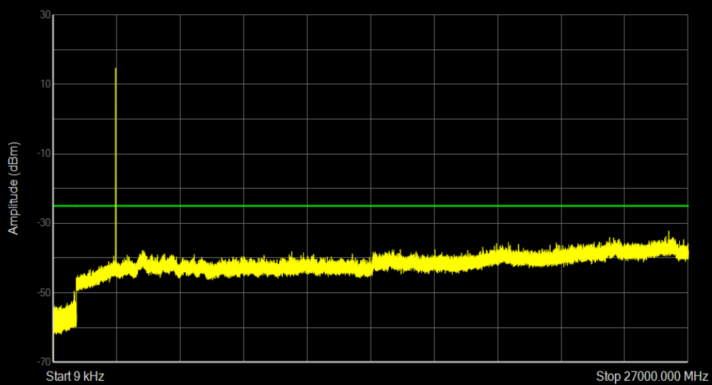
n41 SCS=30kHz CP_QPSK BW=20MHz Channel=535998 RB=1@0
