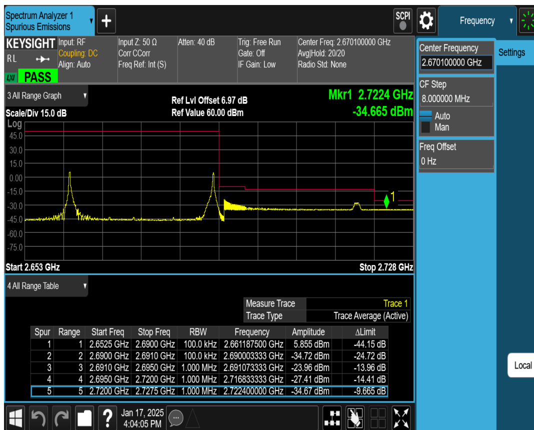
41C 16QAM PCC BW=10MHz Ch=41346 RB=50@0,SCC BW=20MHz Ch=41490 RB=100@0
