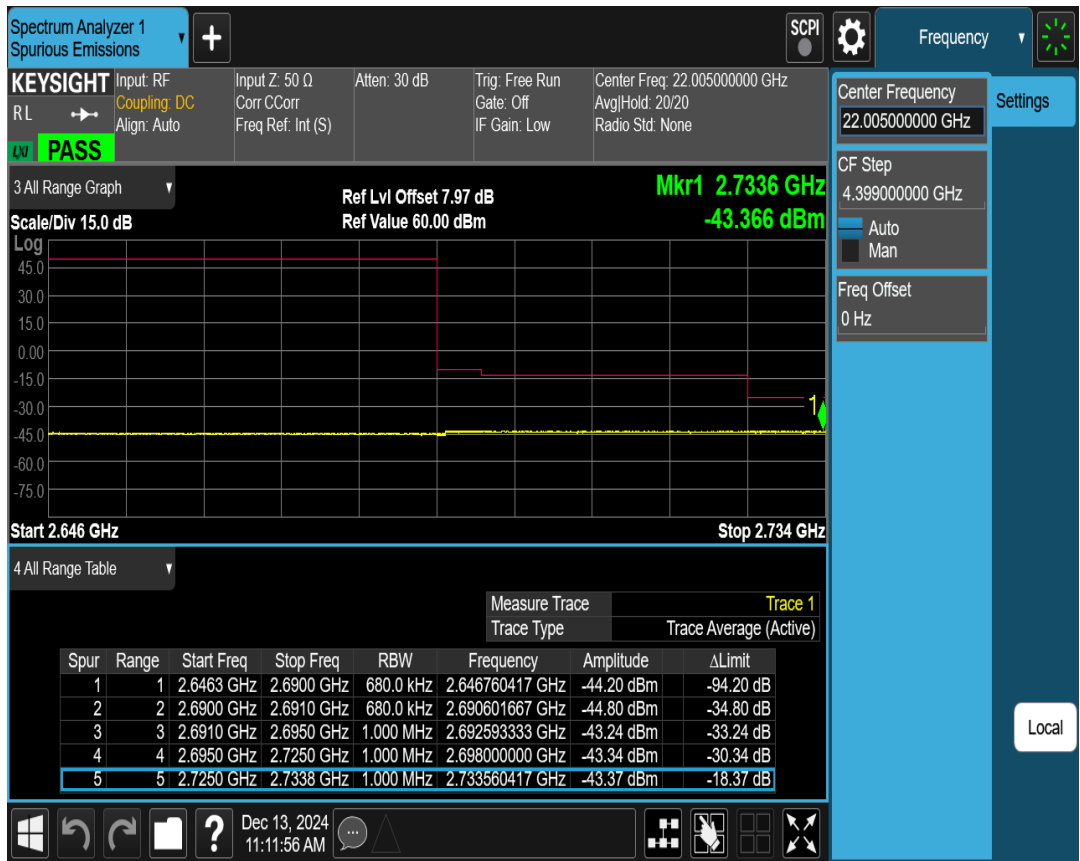
41C 16QAM PCC BW=20MHz Ch=41391 RB=100@0,SCC BW=10MHz Ch=41535 RB=50@0
