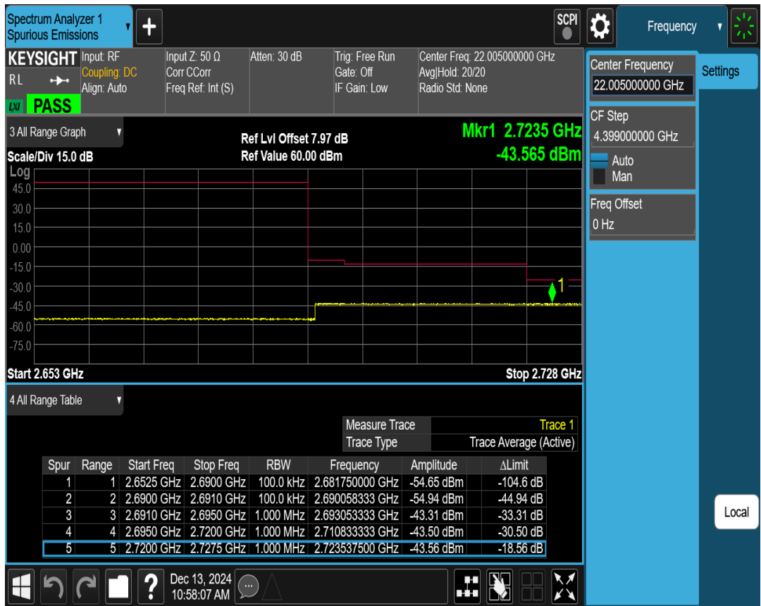
41C QPSK PCC BW=10MHz Ch=41346 RB=50@0,SCC BW=20MHz Ch=41490 RB=100@0
