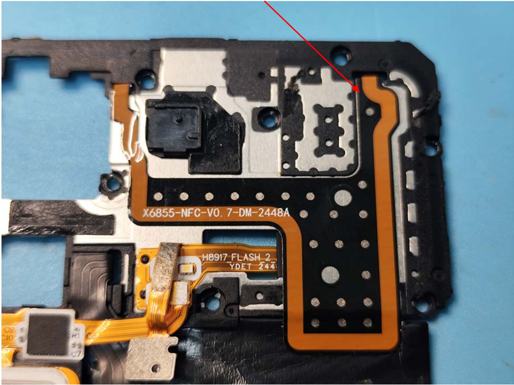
NFC ANT
