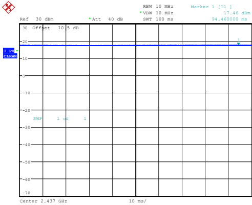
802.11b_2437MHz_Chain 0 100ms,100ms
