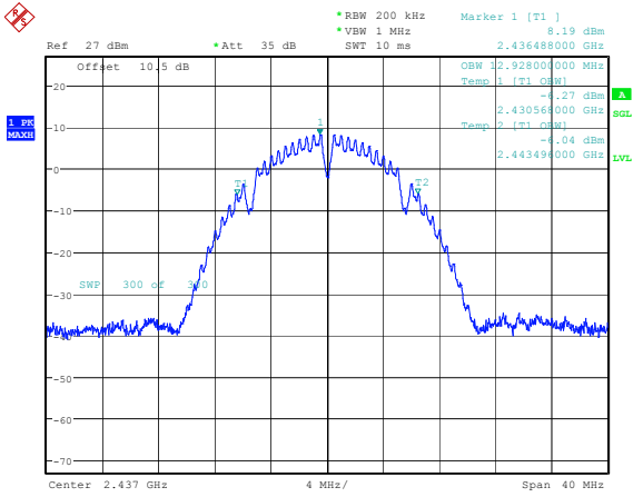
802.11b_2437MHz_Chain 1 12.928MHz
