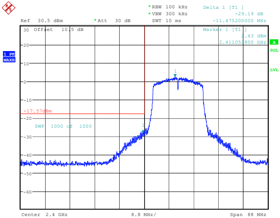
802.11n20_2412MHz_Chain 1 29.19dB
