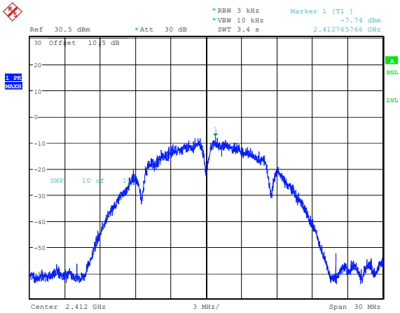
802.11b_2412MHz_Chain 0 -7.74dBm/3kHz
