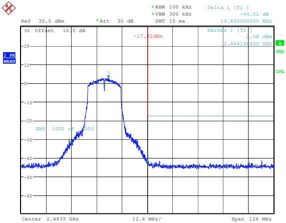
802.11g_2462MHz_Chain 1 44.01dB
