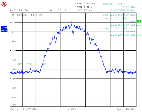
802.11b_2437MHz_Chain 0 12.704MHz
