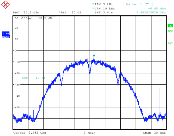
802.11b_2462MHz_Chain 0 -6.05dBm/3kHz
