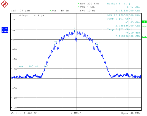
802.11b_2462MHz_Chain 1 12.960MHz
