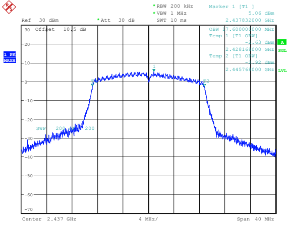
802.11n20_2437MHz_Chain 0 17.600MHz
