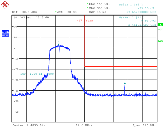
802.11n20_2462MHz_Chain 1 35.10dB
