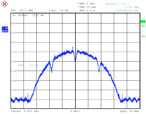
802.11b_2437MHz_Chain 0 -6.87dBm/3kHz
