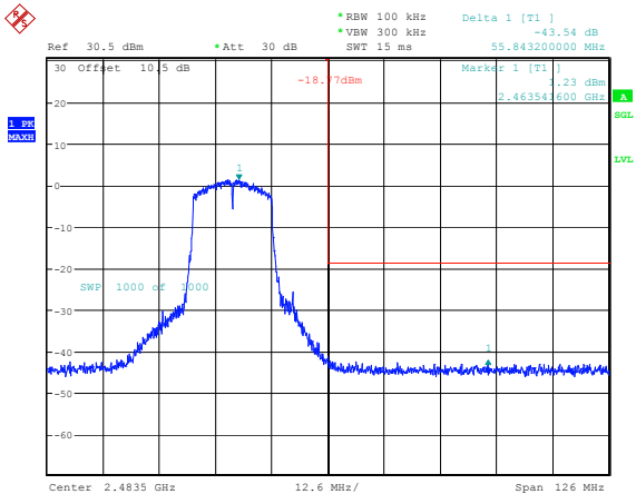
802.11n20_2462MHz_Chain 0 43.54dB
