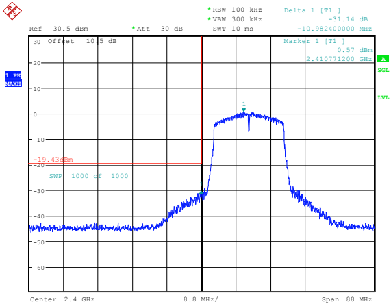
802.11n20_2412MHz_Chain 0 31.14dB
