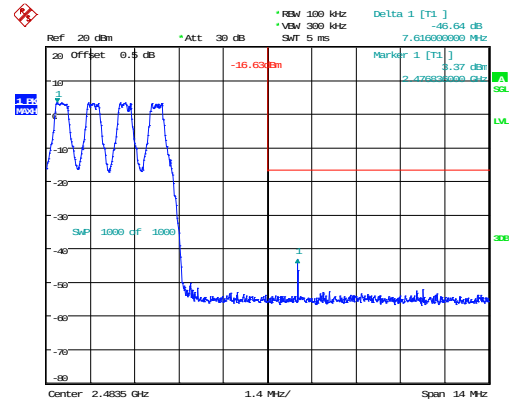
DH1_Hopping_Upper 46.64dB
