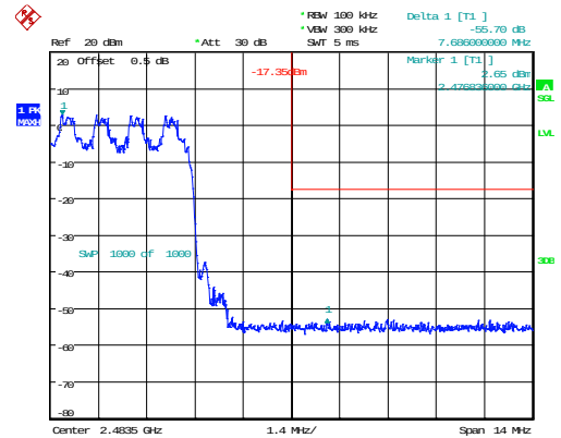
3DH1_Hopping_Upper 55.70dB
