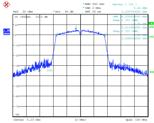
802.11n40_5230MHz 36.200MHz
