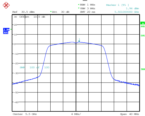
802.11n20_5500MHz
