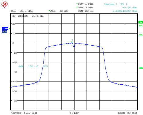
802.11n40_5190MHz
