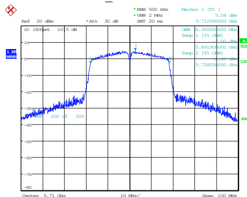
802.11n40 5710MHz 36.300MHz
