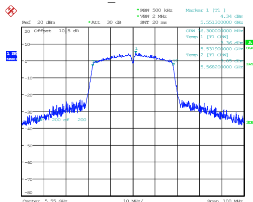
802.11n40 5550MHz 36.300MHz
