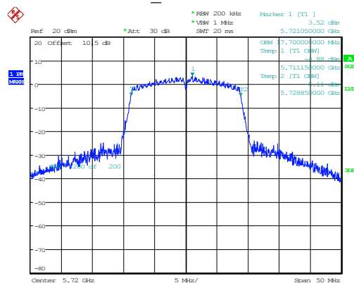
802.11n20 5720MHz 17.700MHz
