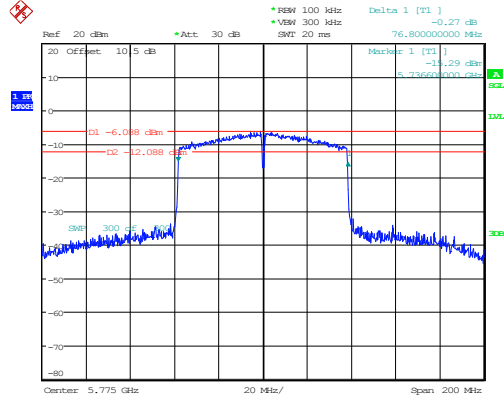
802.11ac80_5775MHz 76.800MHz
