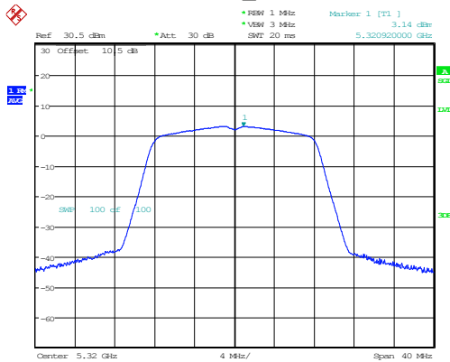
802.11a_5320MHz
