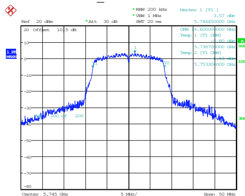
802.11a 5745MHz 16.600MHz
