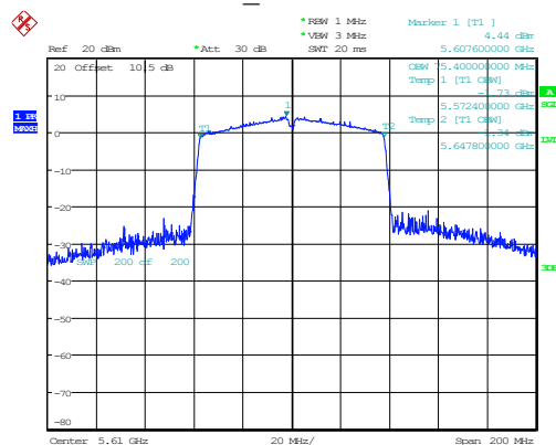
802.11ac80 5610MHz 75.400MHz
