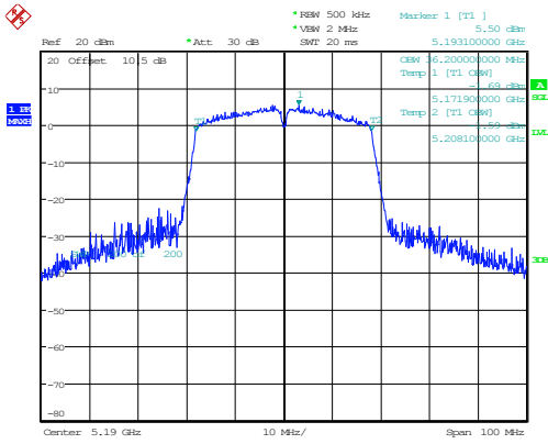
802.11n40_5190MHz 36.200MHz
