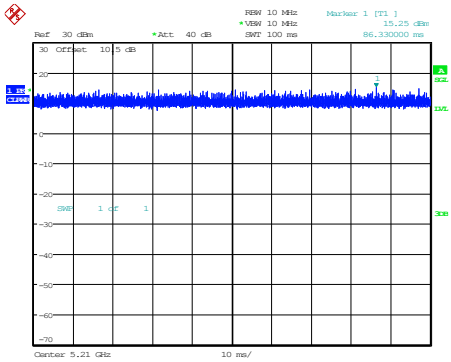
802.11ac80_5210MHz 100ms,100ms
