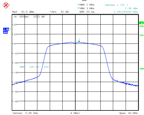
802.11n20_5580MHz
