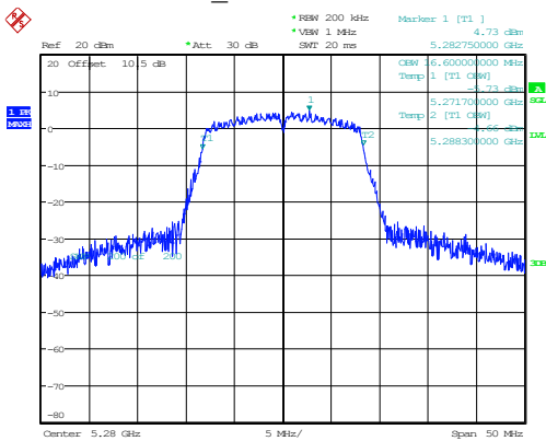
802.11a_5280MHz 16.600MHz
