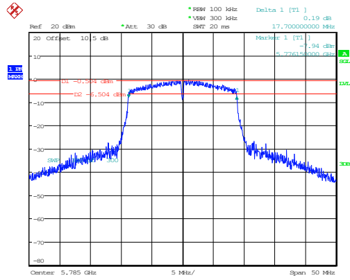
802.11n20_5785MHz 17.700MHz
