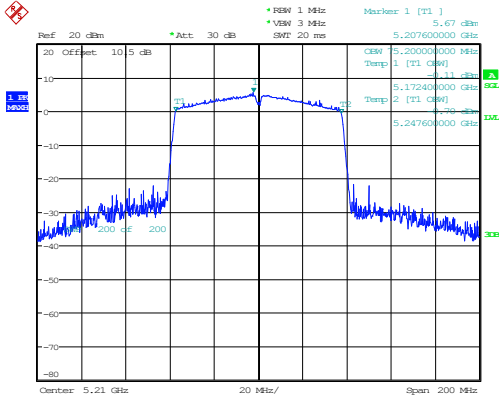
802.11ac80_5210MHz 75.200MHz
