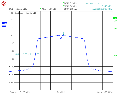
802.11n40_5230MHz
