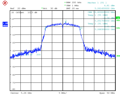
802.11a_5260MHz 16.600MHz
