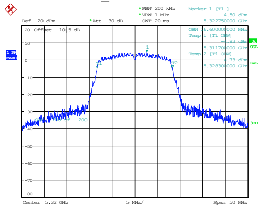
802.11a_5320MHz 16.600MHz
