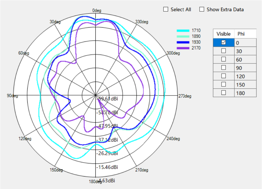
DCS1800/PCS1900/WCDMA B1/B2/B4/LTE B1/2/3/4 Phi=0deg
