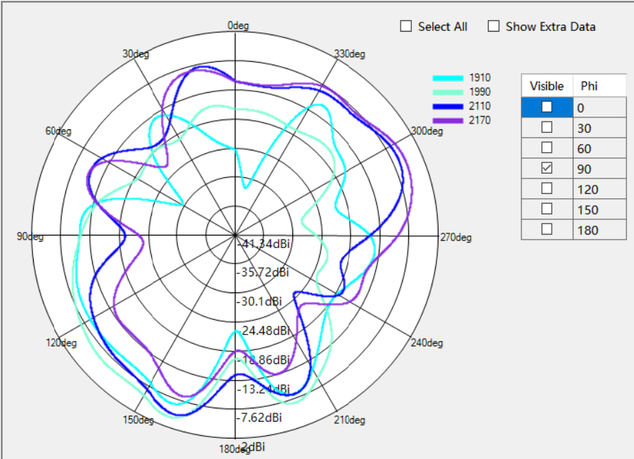
LTE B1Phi=90deg
