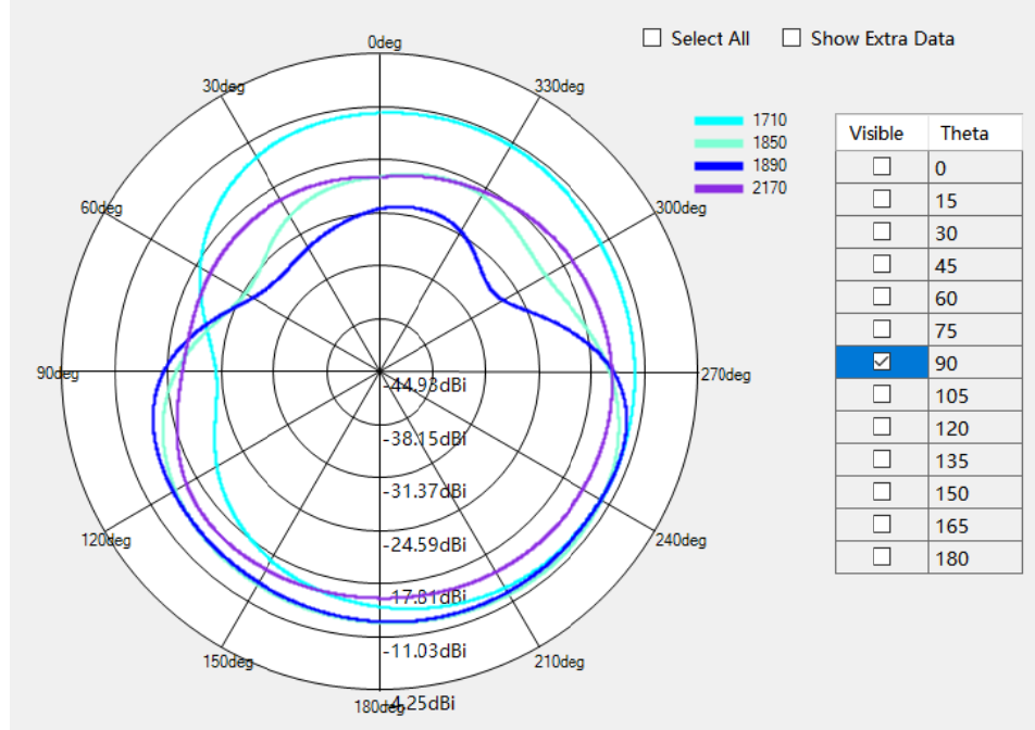
LTE B2/3 Theta=90deg
