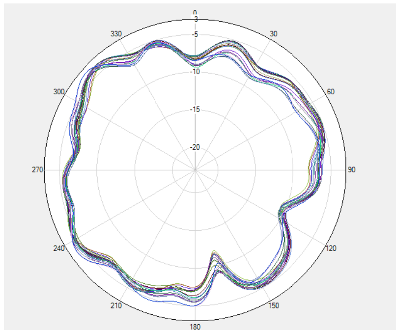
GPS Phi=90deg
