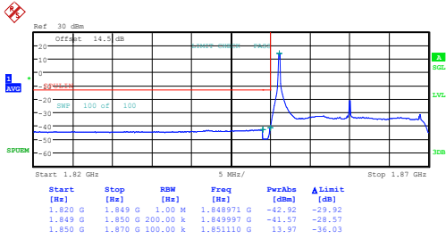
20MHz_Low_QPSK_1@0
