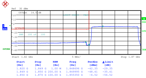
20MHz_Low_QPSK_100@0
