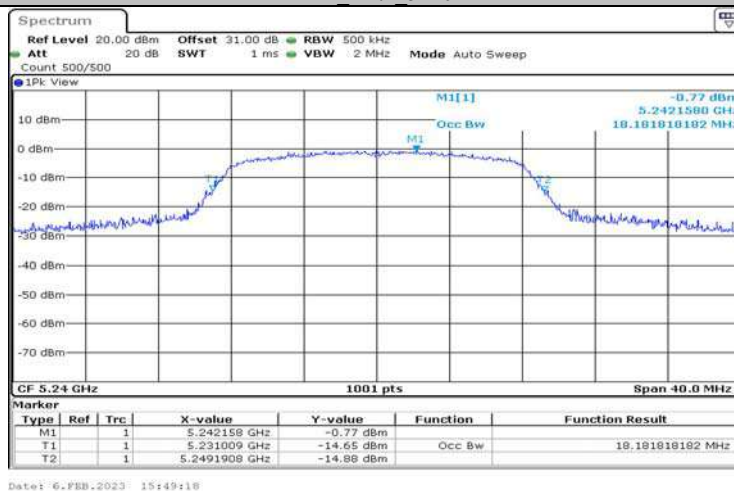
11A_Ant2_5240
