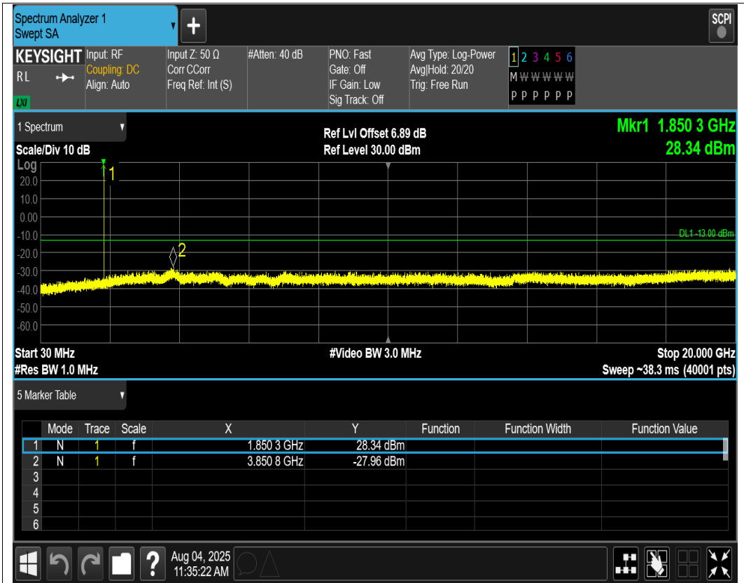
GPRS1900 Channel=512
