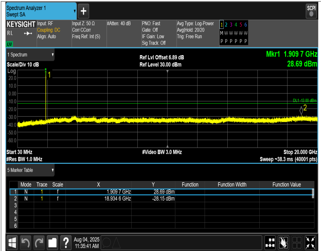
GPRS1900 Channel=810
