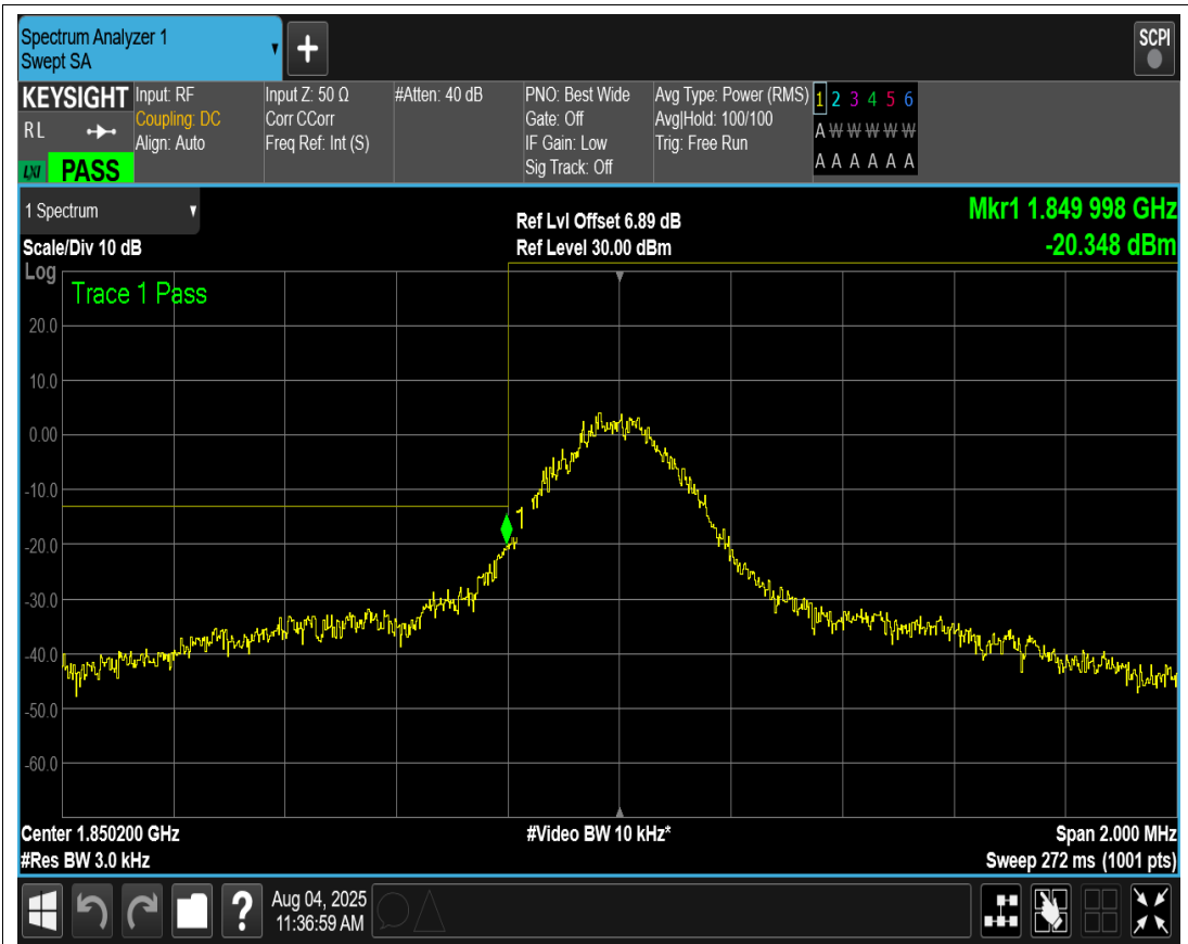
EGPRS1900 Channel=512
