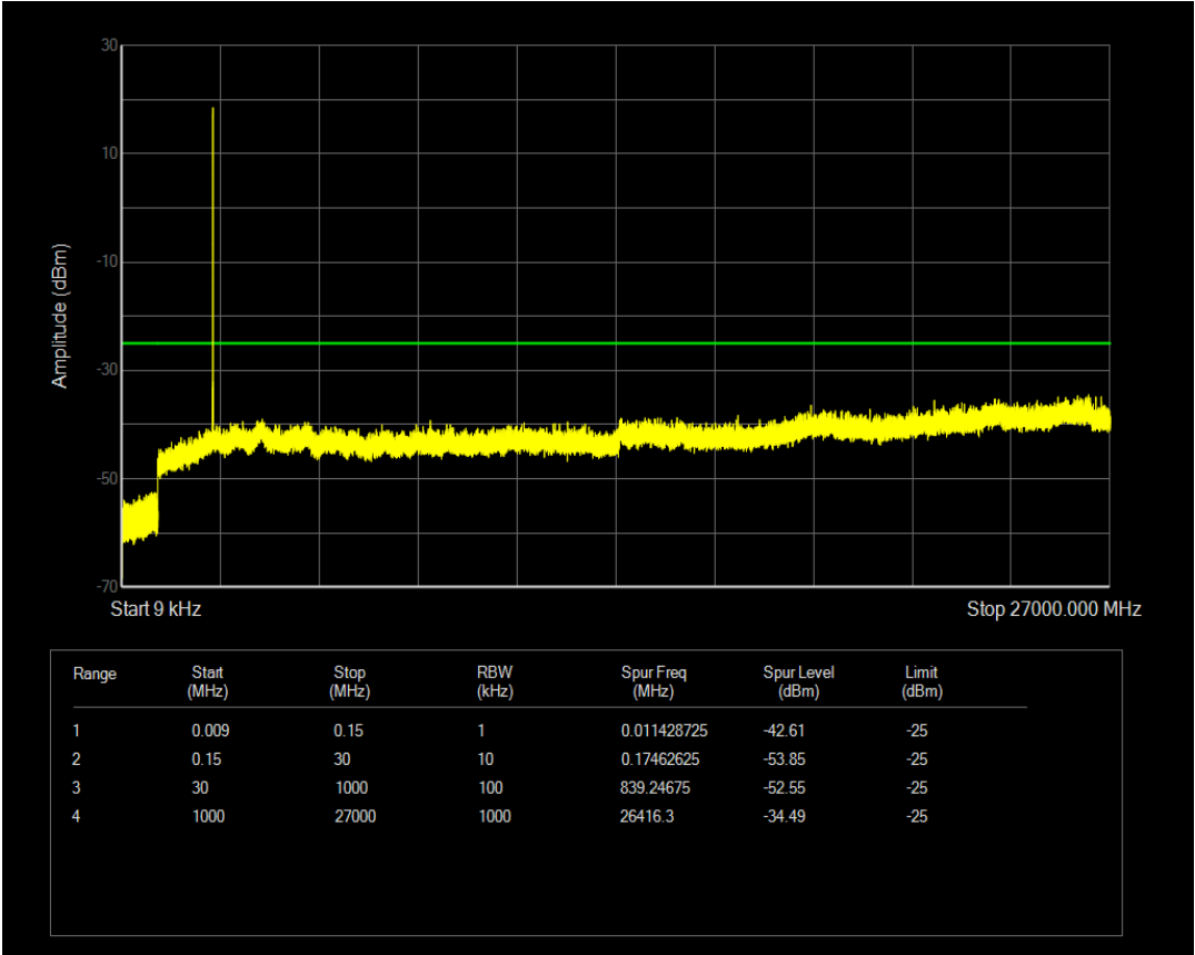
n7 SCS=30kHz CP_QPSK BW=10MHz Channel=501000 RB=1@0
