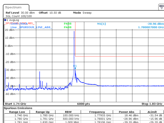
n66_40MHz_15kHz_1760MHz_DFT-s-OFDM QPSK_RB1@215
