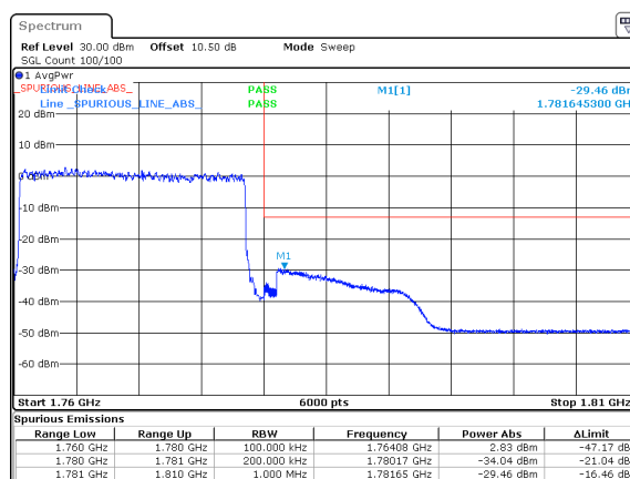
n66_20MHz_15kHz_1770MHz_DFT-s-OFDM QPSK_RB100@0
