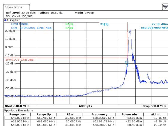
n71_5MHz_15kHz_665.5MHz_DFT-s-OFDM QPSK_RB1@0
