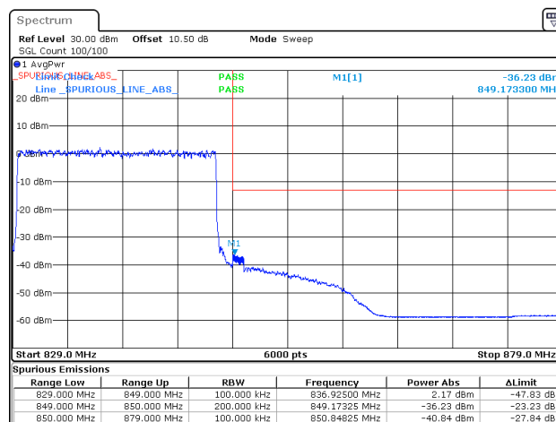
n5_20MHz_15kHz_839MHz_DFT-s-OFDM QPSK_RB100@0
