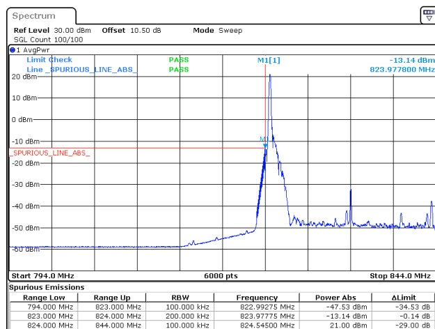
n5_20MHz_15kHz_834MHz_DFT-s-OFDM QPSK_RB1@0
