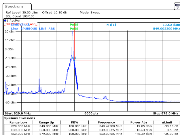
n5_20MHz_15kHz_839MHz_DFT-s-OFDM QPSK_RB1@105
