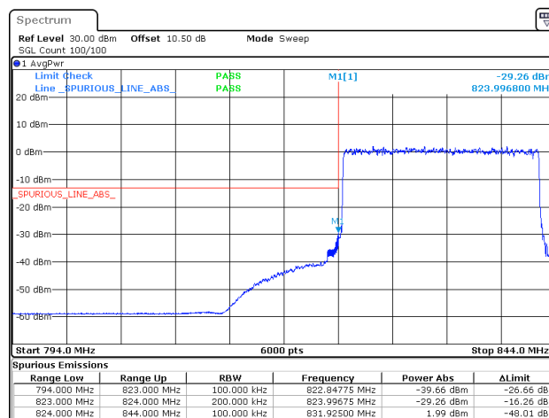
n5_20MHz_15kHz_834MHz_DFT-s-OFDM QPSK_RB100@0
