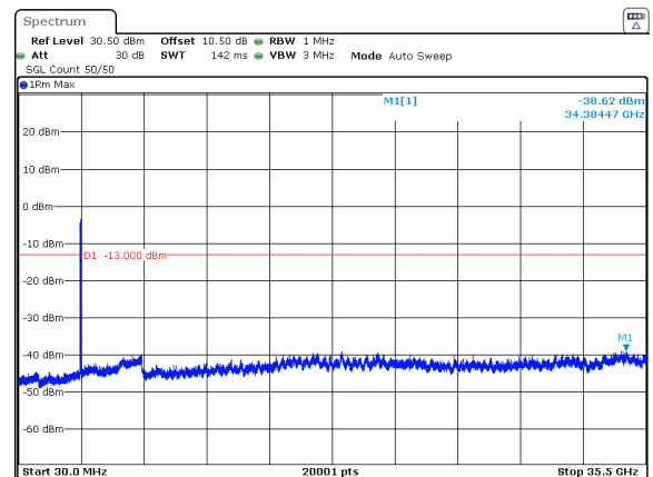
n78_1_80MHz_30kHz_3510MHz_DFT-s-OFDM QPSK_RB216@0 -38.62dBm
