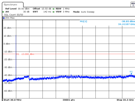
n78_1_80MHz_30kHz_3510MHz_DFT-s-OFDM QPSK_RB1@216 -38.83dBm
