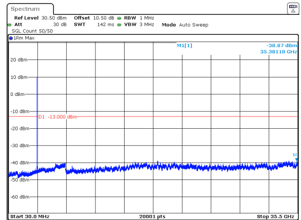
n78_1_80MHz_30kHz_3510MHz_DFT-s-OFDM QPSK_RB1@0 -38.87dBm
