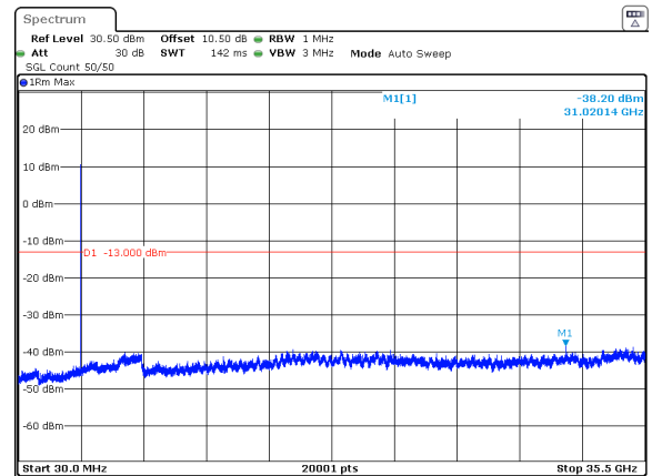
n78_1_80MHz_30kHz_3500MHz_DFT-s-OFDM QPSK_RB1@216 -38.20dBm
