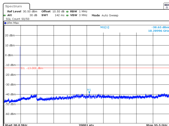
n78_1_15MHz_30kHz_3457.5MHz_DFT-s-OFDM QPSK_RB1@0 -38.65dBm
