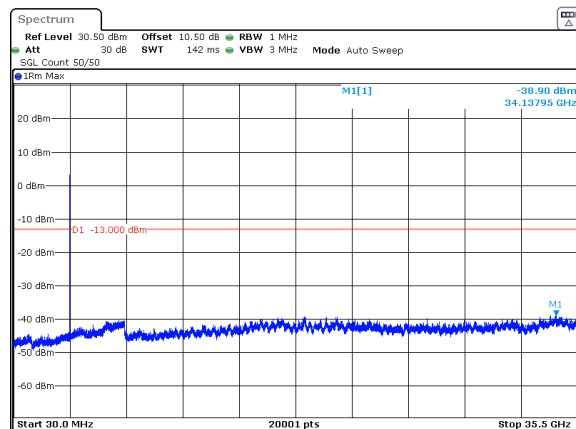
n78_1_15MHz_30kHz_3542.5MHz_DFT-s-OFDM QPSK_RB36@0 -38.90dBm
