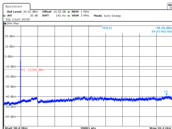
n78_1_15MHz_30kHz_3457.5MHz_DFT-s-OFDM QPSK_RB1@37 -38.58dBm
