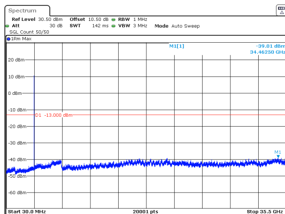
n78_1_15MHz_30kHz_3542.5MHz_DFT-s-OFDM QPSK_RB1@37 -39.01dBm
