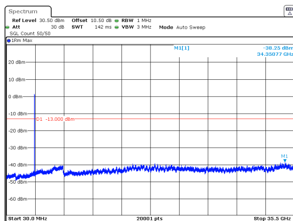
n78_1_20MHz_30kHz_3460MHz_DFT-s-OFDM QPSK_RB1@50 -38.72dBm n78_1_20MHz_30kHz_3460MHz_DFT-s-OFDM QPSK_RB50@0 -38.25dBm
