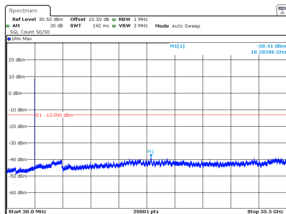
n78_1_15MHz_30kHz_3542.5MHz_DFT-s-OFDM QPSK_RB1@0 -38.41dBm
