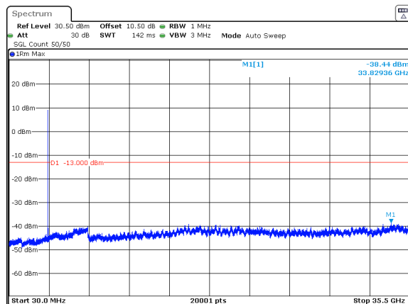
n78_1_20MHz_30kHz_3460MHz_DFT-s-OFDM QPSK_RB1@0 -38.44dBm
