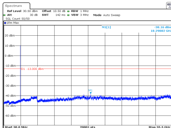
n78_1_15MHz_30kHz_3500MHz_DFT-s-OFDM QPSK_RB1@0 -38.16dBm
