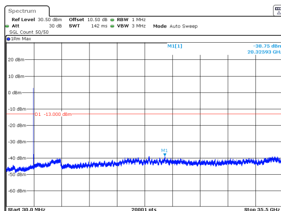
n78_1_15MHz_30kHz_3500MHz_DFT-s-OFDM QPSK_RB1@37 -38.73dBm n78_1_15MHz_30kHz_3500MHz_DFT-s-OFDM QPSK_RB36@0 -38.75dBm
