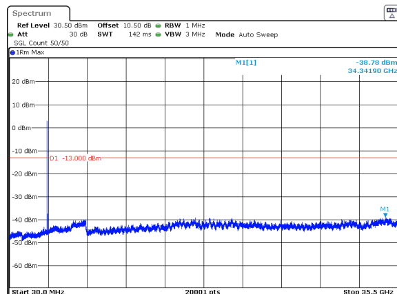
n78_1_15MHz_30kHz_3457.5MHz_DFT-s-OFDM QPSK_RB36@0 -38.78dBm
