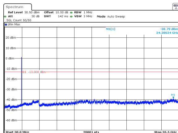
n77_1_20MHz_30kHz_3460MHz_DFT-s-OFDM QPSK_RB50@0 -38.79dBm
