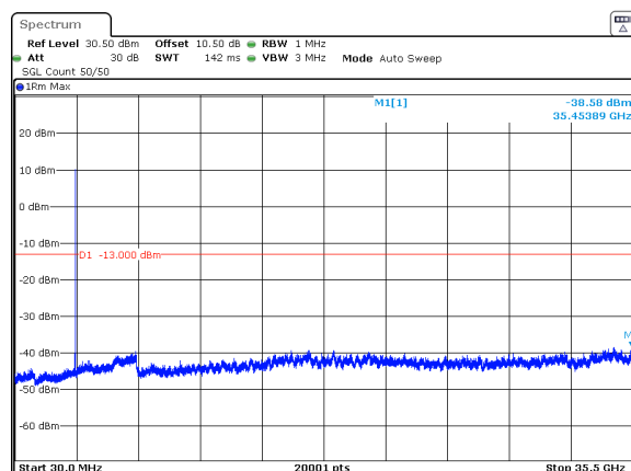
n77_1_20MHz_30kHz_3460MHz_DFT-s-OFDM QPSK_RB1@50 -38.58dBm
